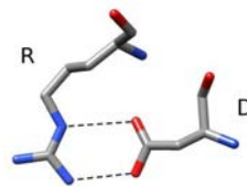
FIGURE 1.9 – Ponts salins entre une arginine (R) et un aspartate (D)
