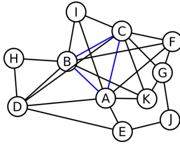
FIGURE 5.4 – Détection d'une graine (ABC, en bleu) dans un graphe non-orienté.
