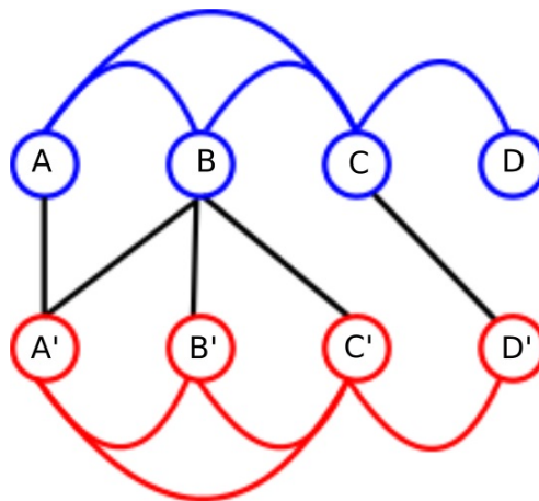
FIGURE 5.1 – Exemple d'alignement k to k , les sommets des pseudocliques (bleu et rouge) se lient pour certains avec plus d'un sommet. Le sommet B est associé aux sommets A', B', C' .
