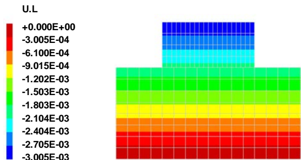
Figure A.2. Déplacement du problème 'patchtest' avec la formulation de pénalisation
