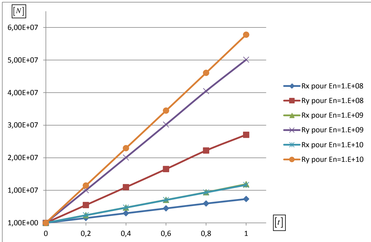
Figure 2.13. Variation de la réaction normale et tangentielle en fonction de la valeur du coefficient de pénalité
