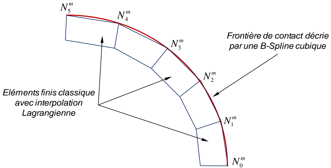
Figure 3.9. Éléments de frontière lissée avec un B-Spline Cubique
