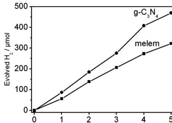
Figure 16 : évolution de la production de \text{H}_2 dans une solution aqueuse à 10%vol de méthanol pour le melem avec 1%Pt et le g-CN avec 1%Pt sous irradiation d'une lampe Xe ( \lambda > 300\text{ nm} ) [73]
