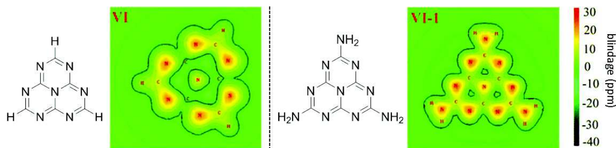
Figure 47 : Cartes de surfaces d'isoblindage ( \text{ICSS}_{zz} ) à 1 Å au-dessus du plan de la molécule pour la heptazine et le melem [37]
