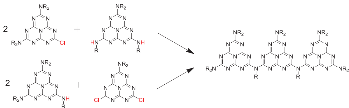
Schéma 29 : voies envisagées pour la synthèse de trimères linéaires
