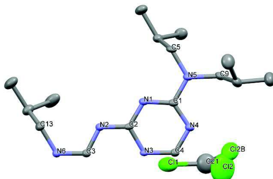
Figure 25 : représentation Mercury [11] de l'unité asymétrique de 1a d'après la diffraction des rayons X avec des ellipsoïdes à 50% de probabilité (atomes d'hydrogène masqués pour une meilleure lisibilité).
