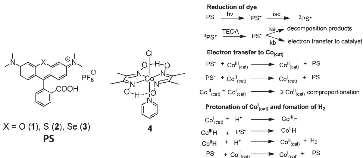
Figure 6 : réaction de formation de \text{H}_2 à partir d'eau, en présence d'un dérivé de rhodamine et d'un complexe de cobalt [16]
