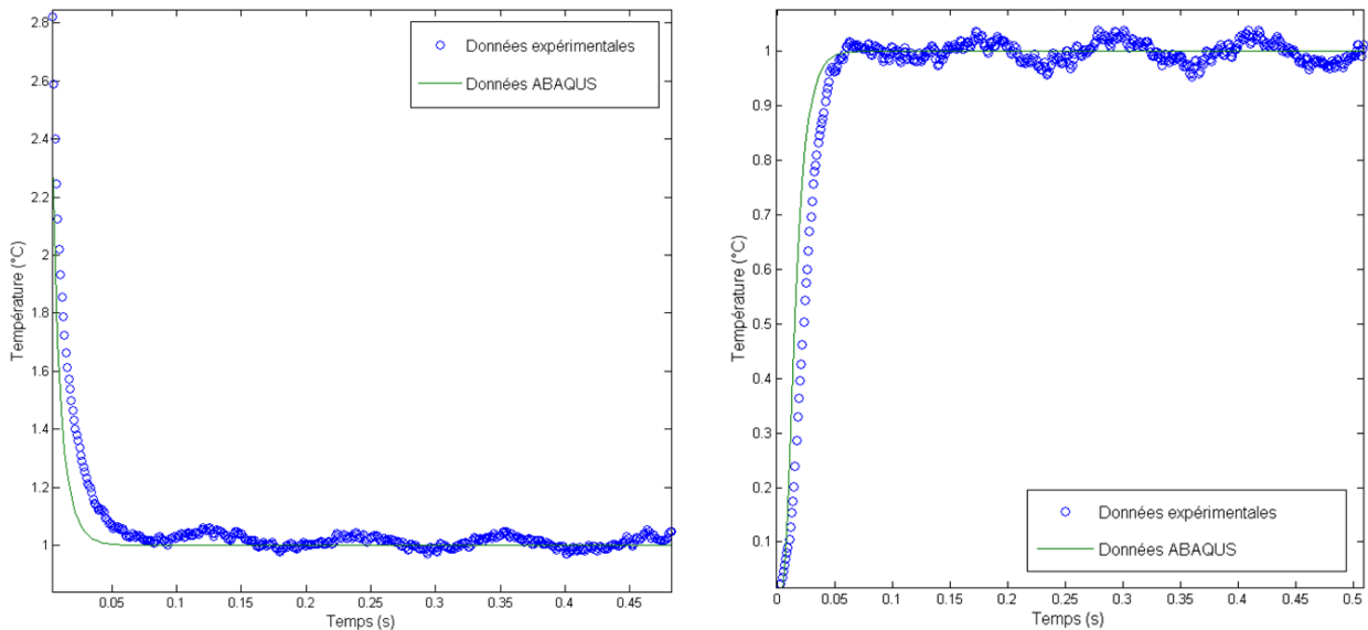
FIGURE 4.28 – Confrontation des thermogrammes expérimentaux et simulés en face avant (gauche) et face arrière (droite)
