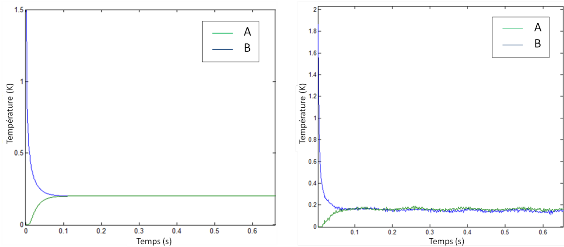
FIGURE 2.12 – Thermogrammes simulés (gauche) et expérimentaux (droite) d’expériences face arrière (A) et face avant (B) sur SiC monolithique tubulaire
