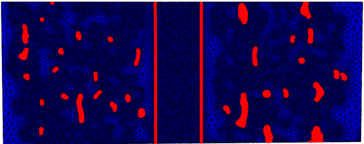
FIGURE 4.40 – Prise en compte dans le maillage d'une résistance thermique de contact entre les couches de la gaine sandwich
