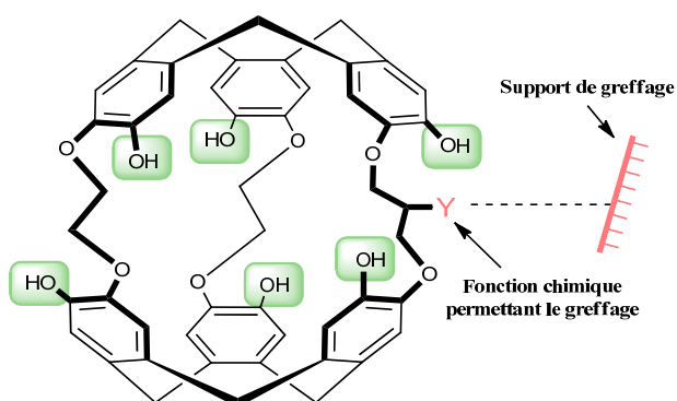
Figure 53 : Cible synthétique pour la complexation des cations \text{Cs}^+ et \text{Tl}^+ .
