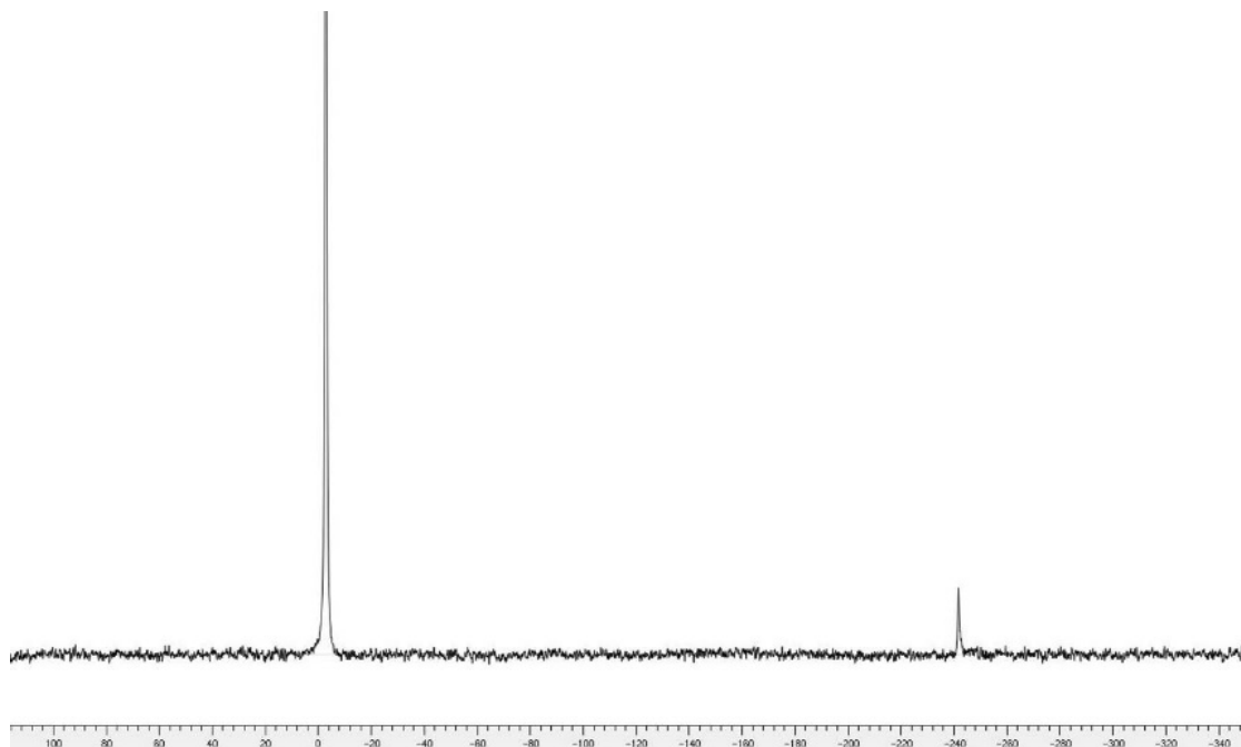
Figure 127 : Spectre RMN du noyau de césium ^{133}\text{Cs} enregistré à 298 K pour une solution de NaOD/ \text{D}_2\text{O} contenant le cryptophane 1 et une faible quantité de CsOH.
