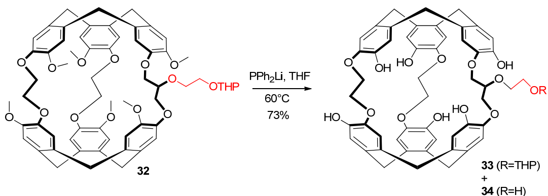
Figure 77 : Réaction de déméthylation du cryptophane 32 menant à un mélange des cryptophane 33 et 34 présentant une fonction alcool protégée ou non.
