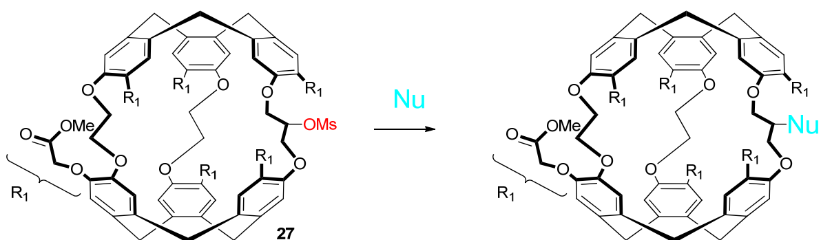
Figure 71 : Illustration des essais d'alkylation entre le cryptophane 27 et des nucléophiles Nu .
