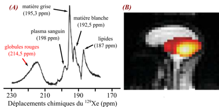
Figure 28 : (A) : Spectre RMN du cerveau d'un sujet humain en bonne santé ayant inhalé du xénon hyperpolarisé. (B) : Image obtenue du même sujet en sélectionnant la fréquence correspondant au 129 Xe dans les globules rouges. 63
