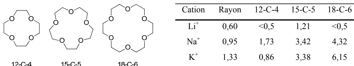
Figure 3 : À gauche : les structures de trois éthers couronnes de tailles différentes. À droite : tableau récapitulatif des rayons des cations complexés et les constantes d'association (exprimées en log K a ) pour les différents éthers couronnes.
