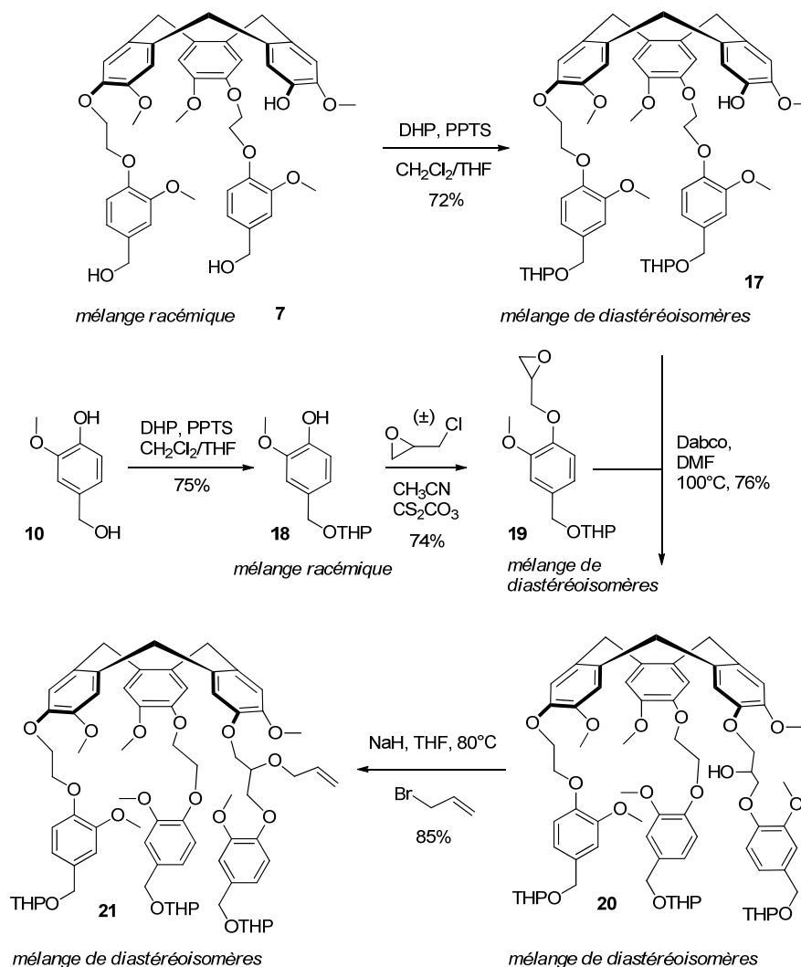
Figure 59 : Schéma de synthèse du composé tripointé 21 sous la forme d'un mélange de diastéréoisomères.
