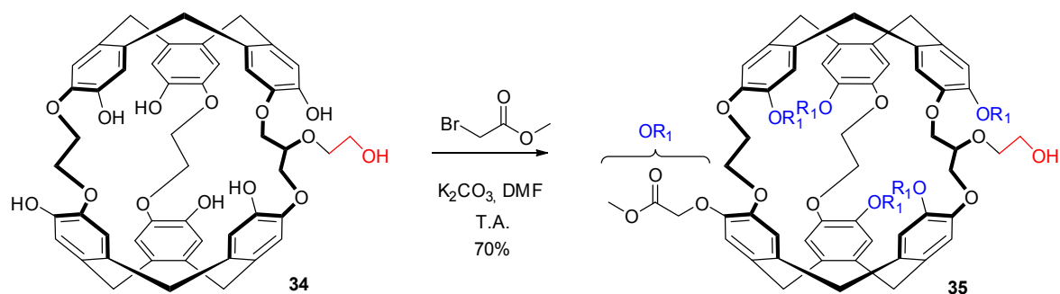
Figure 78 : Alkylation des phénols du composé 34 par le bromoacétate de méthyle pour mener au cryptophane hexaester 35 .
