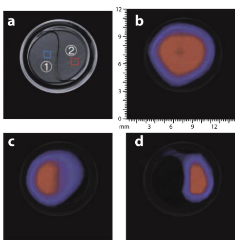
Figure 32 : (a) Tube tapissé d'un lit d'agarose/avidine divisé en deux compartiments. La zone 1 ne contient pas de biosonde alors que la zone 2 contient une biosonde à une concentration de 5\mu\text{M} . (b) Image obtenue par une acquisition hors résonance. (c) Image obtenue lors d'une acquisition en irradiant à la fréquence de résonance du xénon encapsulé dans la biosonde. (d) Résultat de l'expérience HyperCEST obtenue par soustraction des signaux (b) et (c).
