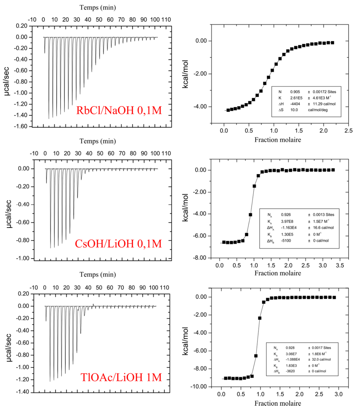
Figure 126 : Enthalpogramme correspondant aux titrages calorimétriques du cryptophane 1 . En haut : solution de 1 à 0,1 nmol.L -1 dans NaOH 0,1 mol.L -1 titrée par ajouts d'une solution de RbCl à 1,0 nmol.L -1 dans NaOH 0,1 mol.L -1 . Au milieu : solution de 1 à 0,03 nmol.L -1 dans LiOH 0,1 mol.L -1 titrée par ajouts d'une solution de CsOH à 0,404 nmol.L -1 et RbCl à 0,302 mol.L -1 dans LiOH 0,1 mol.L -1 . En bas : solution de 1 à 0,03 nmol.L -1 dans LiOH 1 mol.L -1 titrée par ajouts d'une solution de TIOAc à 0,395 nmol.L -1 et RbCl à 0,499 mol.L -1 dans LiOH 1 mol.L -1 .
