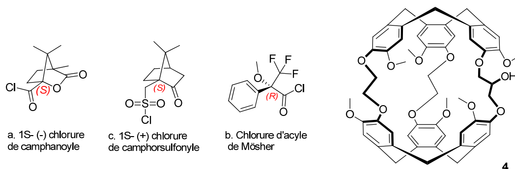
Figure 115 : Exemple d'agents de dédoublement courants pour la séparation des mélanges racémique des alcools et structure du cryptophane 4.
