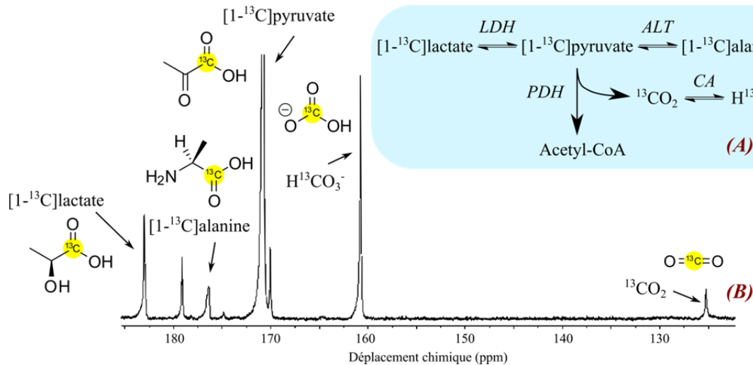
Figure 26 : (A) Diagramme du métabolisme du pyruvate décrivant sa transformation par les enzymes LDH , ALT et PDH pour donner respectivement comme produit le lactate, l'alanine et le \text{CO}_2 . Ce dernier est par la suite transformé en hydrogénocarbonate par l'anhydrase carbonique ( CA ). (B) Spectre RMN ^{13}\text{C} enregistré en 1 scan à partir d'un cœur de rat dans lequel a été injecté du [1-^{13}\text{C}] pyruvate hyperpolarisé. On peut identifier sur ce spectre tous les produits issus du métabolisme présenté. 62,64
