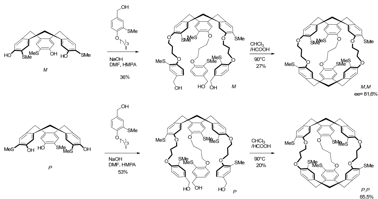
Figure 107 : Synthèse de deux cryptophanes soufrés énantiomériquement enrichis à partir des CTB énantiopurs.
