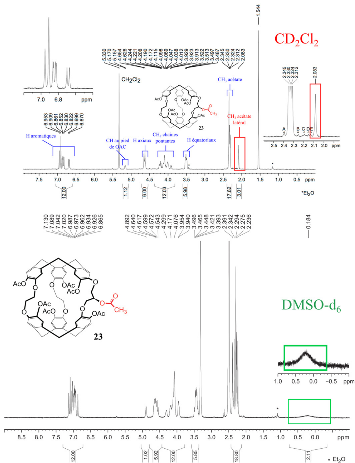
Figure 62 : Spectres RMN 1 H du composé 23 à 298 K. En haut : spectre enregistré dans le CD 2 Cl 2 , le signal du groupement méthyle de l'acétate porté par la chaîne pontante est alors fin et autour de 2,08 ppm. En bas : spectre enregistré dans le DMSO-d 6 , le signal du même groupement méthyle est à présent beaucoup plus large et se trouve entre 0 et 0,5 ppm.
