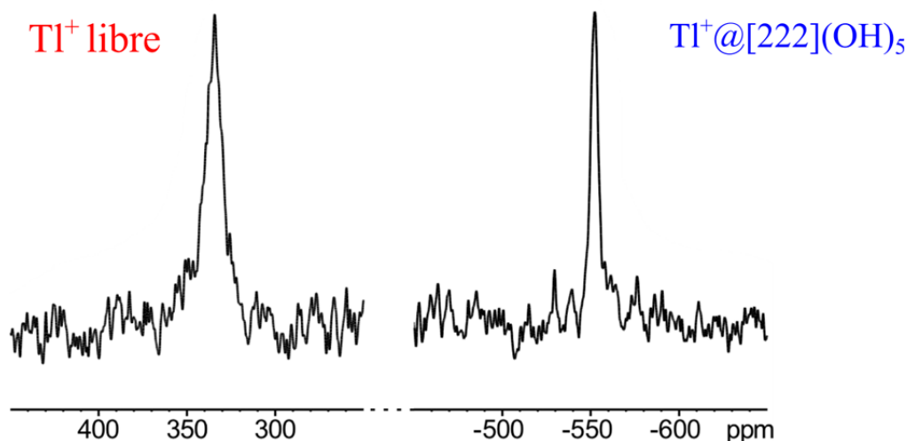
Figure 51 : Spectre RMN du ^{205}\text{Tl} enregistré à 298 K pour le cryptophane [\text{222}](\text{OH})_5 dans une solution de \text{NaOD}/\text{D}_2\text{O} (0,1M) en présence de \text{TlOAc} .
