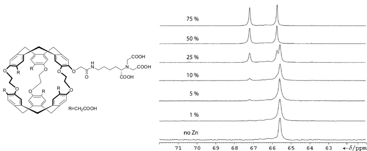
Figure 83 : À gauche : structure de la biosonde comportant la tête NTA. À droite : spectres RMN du ^{129}\text{Xe} enregistrés en un scan pour des ajouts successifs de cation Zn^{2+} à une solution de biosonde à la concentration de 260 \mu\text{M} . Seule la partie présentant le signal du xénon encapsulé dans le cryptophane est montrée sur ces spectres RMN. 102
