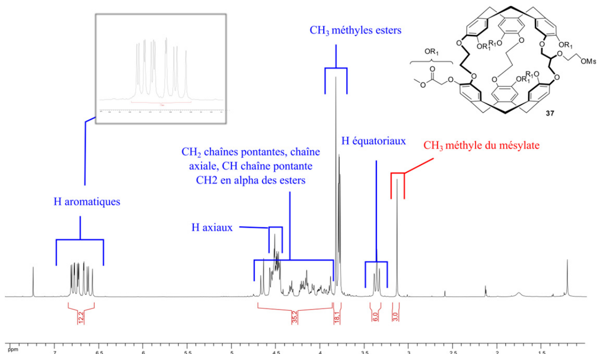
Figure 82 : Spectre RMN 1 H du composé 37 enregistré à 500 MHz.
