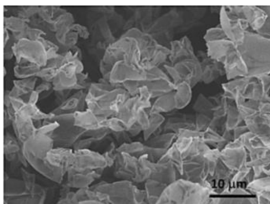
Figure 126: Image MEB d'une électrode composé de feuillets de graphène [400]
