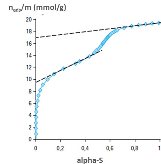
Figure 9: Courbe transformée alpha-S d'un charbon microporeux [29]
