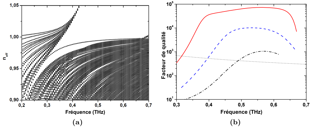
FIGURE 3.41 – Diagramme des indices effectifs du guide dont le cristal à BIP est composé de 4 anneaux de tiges de silice de 200\ \mu\text{m} de diamètre et régulièrement espacées de 1,8\ \text{mm} , soit d/\Lambda = 0,11 (a), influence du ratio d/\Lambda de ce même guide sur le facteur de qualité, en fonction de la fréquence, avec d/\Lambda = 0,3 (traits noirs discontinus), d/\Lambda = 0,2 (tirets bleus) et d/\Lambda = 0,1 (ligne rouge), en pointillé le facteur de qualité intrinsèque de la silice d'après [4] (b).
