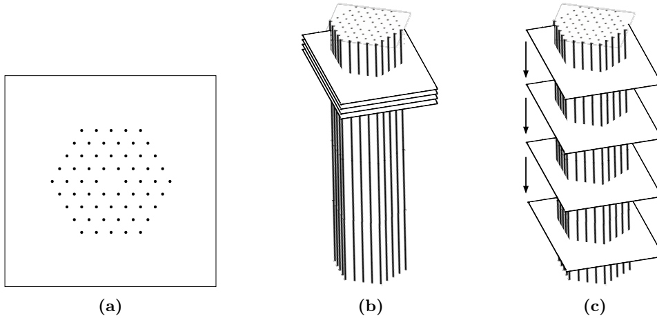
FIGURE 3.42 – Illustration du gabarit de papier (a), illustration du montage une fois que les tiges sont passées dans les trous du gabarit (b), répartition des gabarits de papier pour le maintien des tiges sur toute la longueur du guide réalisé (c).
