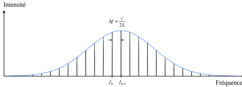
FIGURE 1.19 – Graphique représentant l'allure spectrale de l'intensité d'une l'impulsion laser (en noir) modulée par le gain du milieu actif (en bleu).
