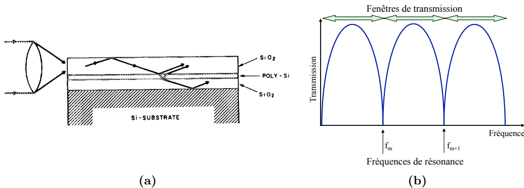
FIGURE 2.6 – (a) Schéma du guide d'onde réalisé par M. A. Duguay et al. [78] et dont le confinement est réalisé dans la couche « SiO 2 » supérieure, par réflexion totale interne au-dessus et par réflexion antirésonante en dessous. (b) Illustration des bandes de transmissions du guide, interrompues par les fréquences de résonances.
