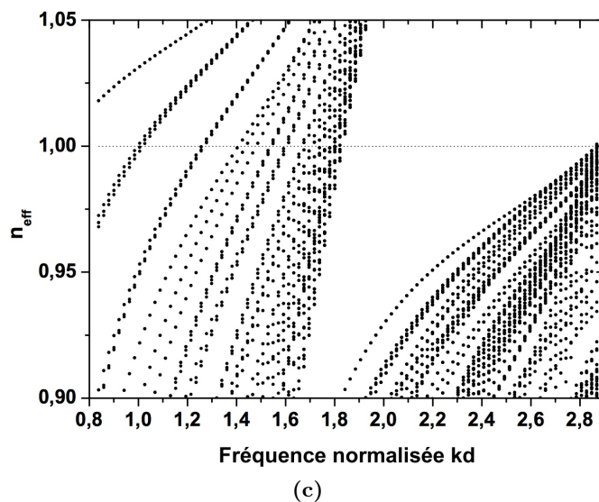
FIGURE 2.37 – Diagramme des indices effectifs de la structure à 3 anneaux avec un rapport d/\Lambda = 0,1 (a), d/\Lambda = 0,2 (b), d/\Lambda = 0,3 (c).
