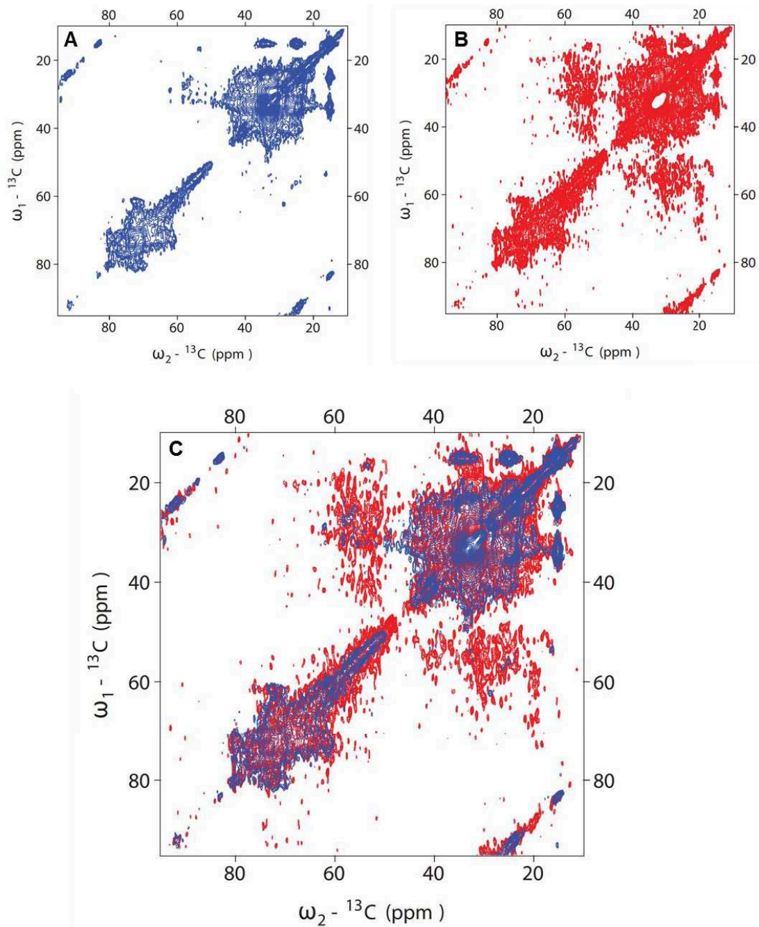
Figure 9. Spectres de corrélation 2D {}^{13}\text{C} - {}^{13}\text{C} DARR obtenus sur des préparations d'enveloppe cellulaires de (U- {}^{13}\text{C} , {}^{15}\text{N} )- E. coli avec ou sans induction de KpOmpA. A. Echantillon non-induit. B. Echantillon Induit. C. Superposition des spectres des échantillons non-induit (A), en bleu, et induit (B), en rouge. L'ensemble des données RMN ont été obtenues sur un spectromètre Bruker Avance III HD opérant à une fréquence de Larmor {}^1\text{H} de 700 MHz et équipé d'une sonde MAS E-Free 3.2 mm (Bruker BioSpin). Les expériences 2D {}^{13}\text{C} - {}^{13}\text{C} DARR ont été enregistrées à une fréquence de rotation de 12 KHz et à une température de +2°C en utilisant un temps de mélange de 50 ms et un temps d'acquisition de 38 heures.
