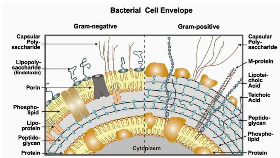
Figure 13. Représentation schématique de l'enveloppe bactérienne, Gram-négative à droite et Gram-positif à gauche. L'enveloppe des bactéries Gram-négatives est constituée d'une couche de peptidoglycane plus fine ainsi que d'une membrane externe absente chez les bactéries Gram-positives. Figure reprise de (Muller-Loennies et al. 2007).
