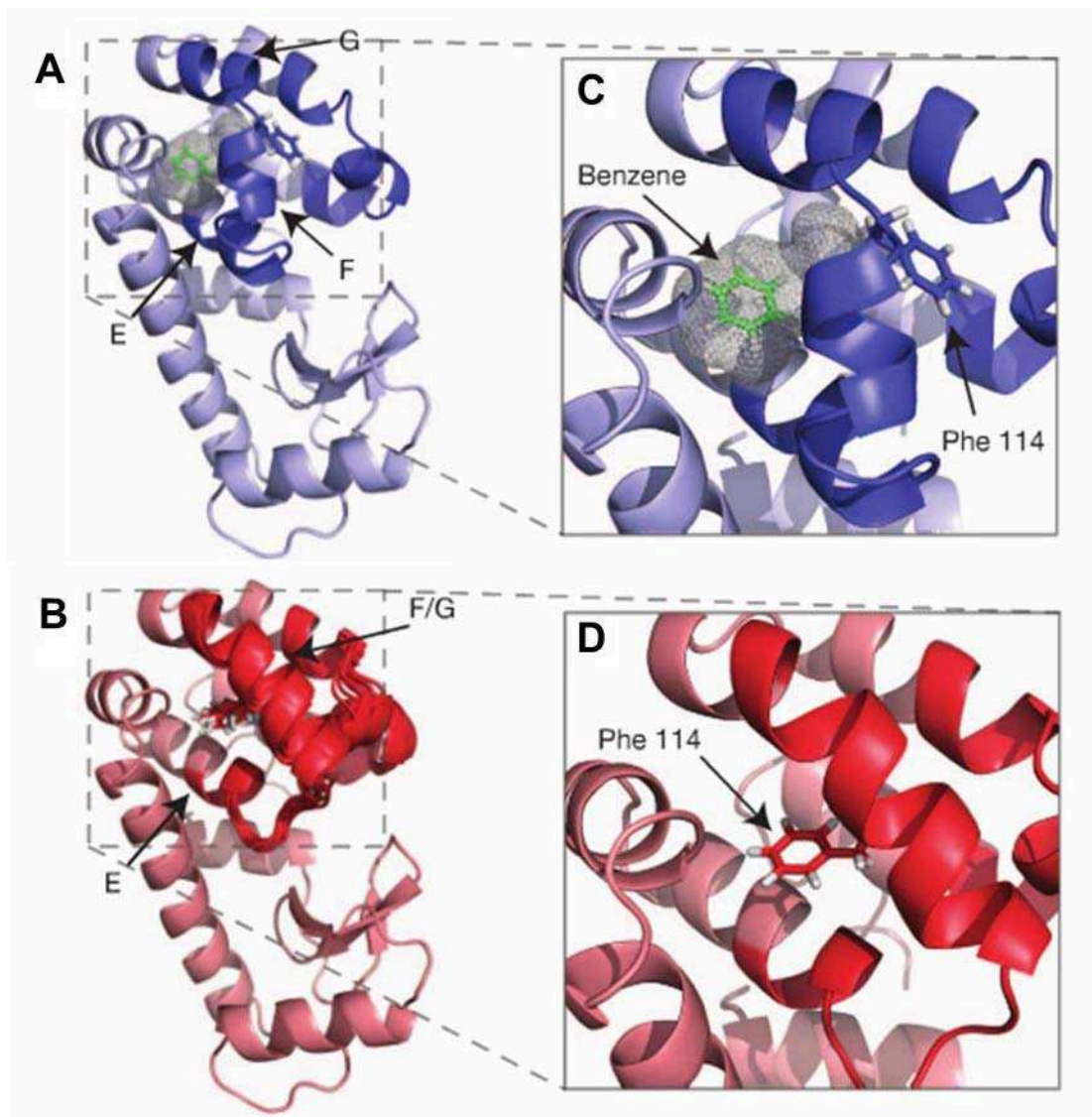
Figure 29. Structure de l'état « invisible » de L99A-T4L. A. Structure cristallographique de l'état de base de L99A-T4L avec une molécule de benzène, en vert, dans la cavité. Les positions des hélices E, F et G sont indiquées ainsi que la chaîne latérale de F114. B. Superposition des 10 structures de plus basse énergie de l'état excité de L99A-T4L. C. et D. Vue rapprochée de la chaîne latérale de F114 dans les structures de l'état basal (C.) et de l'état excité (D.) de L99A-T4L. Adapté de (Bouvignies et al. 2011).
