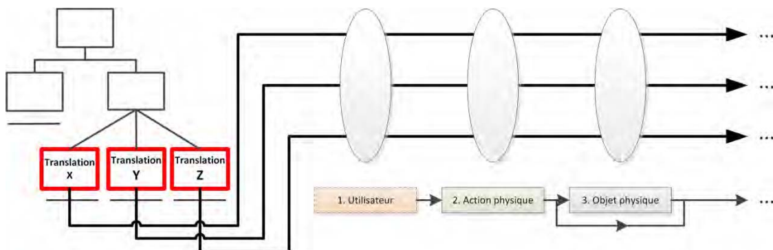
Figure 21 : Illustration avec la notation 3DIM de la propriété d'homogénéité physique avec la valeur haute . Les tâches encadrées en rouge sont similaires.
