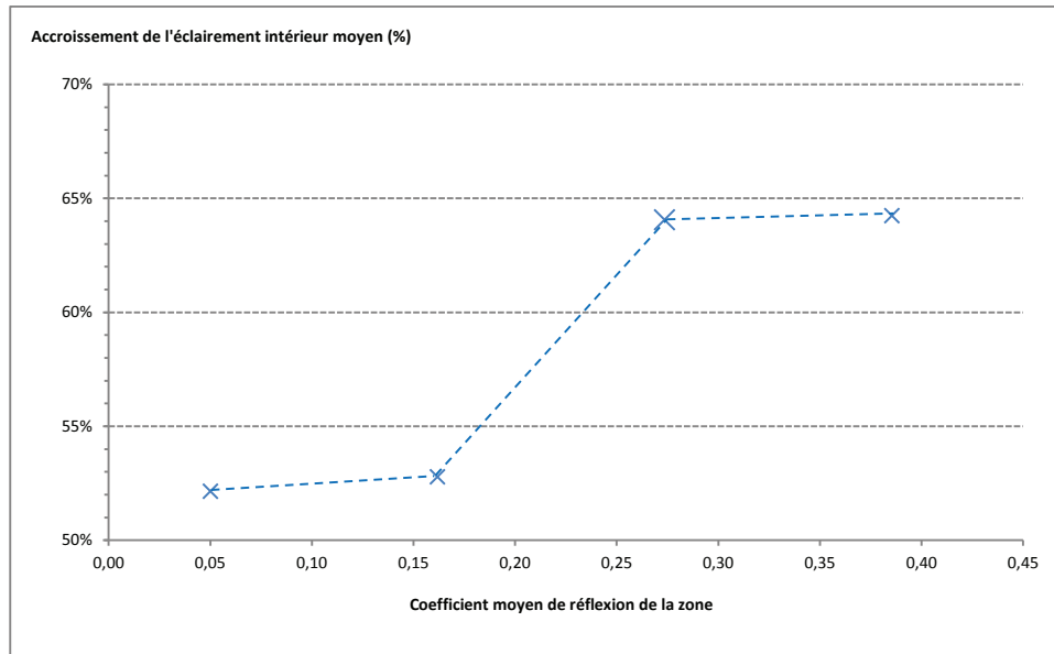
Figure 92 : Évolution de l'éclairement intérieur en fonction du coefficient de réflexion moyen de la zone Cette constatation peut être imagée par la Figure 92. En passant d'une pièce aux parois noires à une pièce aux parois blanches, nous pouvons doubler le niveau d'éclairement intérieur.
