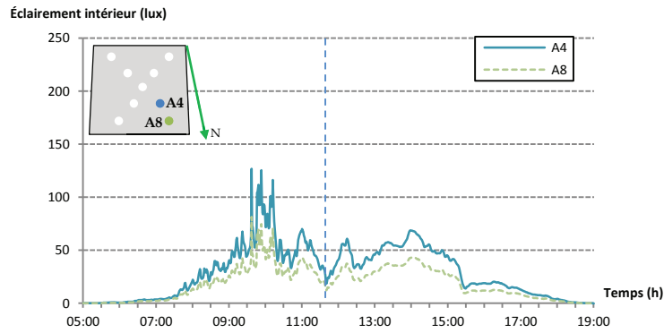
Figure 84 : Évolution horaire des éclairages extérieur et intérieur pour une journée de ciel couvert (30 novembre 2014)
