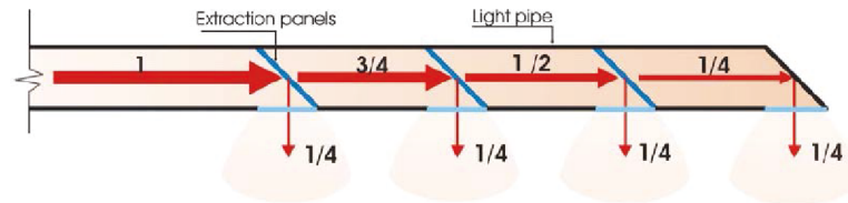
Figure 29 : Principe de l'extraction lumineuse selon Edmonds (Edmonds, Reppel, and Jardine 1997; Hansen 2006)
