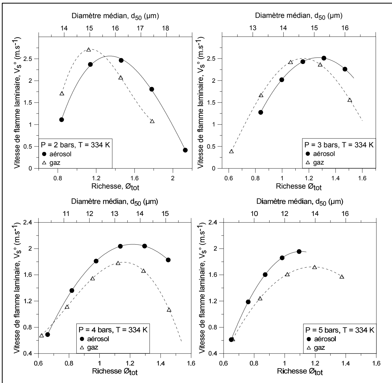
Figure IV. 3 : La vitesse de propagation de la flamme V_s en fonction de la richesse totale et la pression initiale
