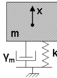
Figure 180: Schéma mécanique équivalent
