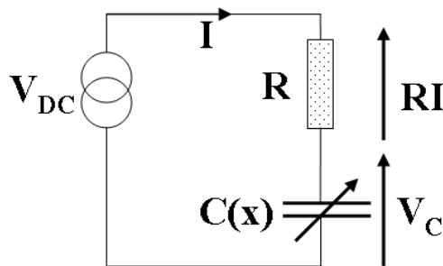
Figure 179: Schéma électrique équivalent
