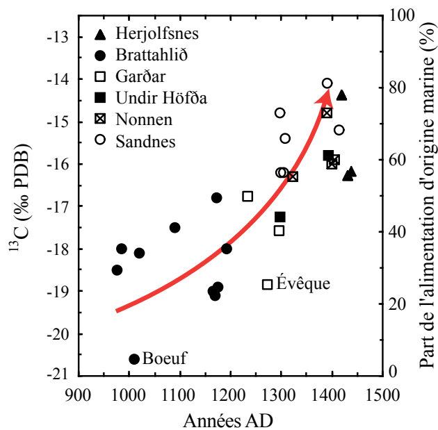
Fig. 2.5 \delta^{13}\text{C} mesuré sur des ossements vikings et exprimé en fonction du temps. Les différents symboles font référence aux cimetières dans lesquels furent inhumés les individus. Celui de Sandnes se trouve dans l'établissement occidental ( Vesterbygden ), les autres se trouvent dans l'établissement oriental ( Østerbygden ). L'axe de droite indique la proportion de produits d'origine marine dans l'alimentation, estimée à partir du \delta^{13}\text{C} . Remarquez la valeur terrestre de l'os de boeuf, un herbivore strict. Le haut statut social associé à un régime alimentaire privilégié ou son arrivée récente de Norvège pourrait expliquer la faible part de marin dans l'alimentation de l'évêque, enterré dans la cathédrale de Garðar . (Modifié, d'après Arneborg et al. , 1999).
