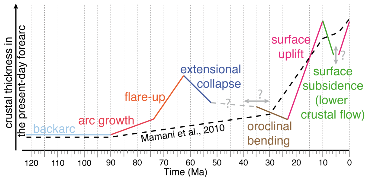
Figure E : Diagramme montrant l'évolution schématique de l'épaisseur crustale de l'avant-arc sud péruvien au cours du temps tel que proposé dans cette thèse (en couleur). L'évolution basée sur les données géochimiques proposée par Mamani et al. (2012) est reportée pour comparaison (ligne noire en pointillés). Pas d'échelle verticale.
