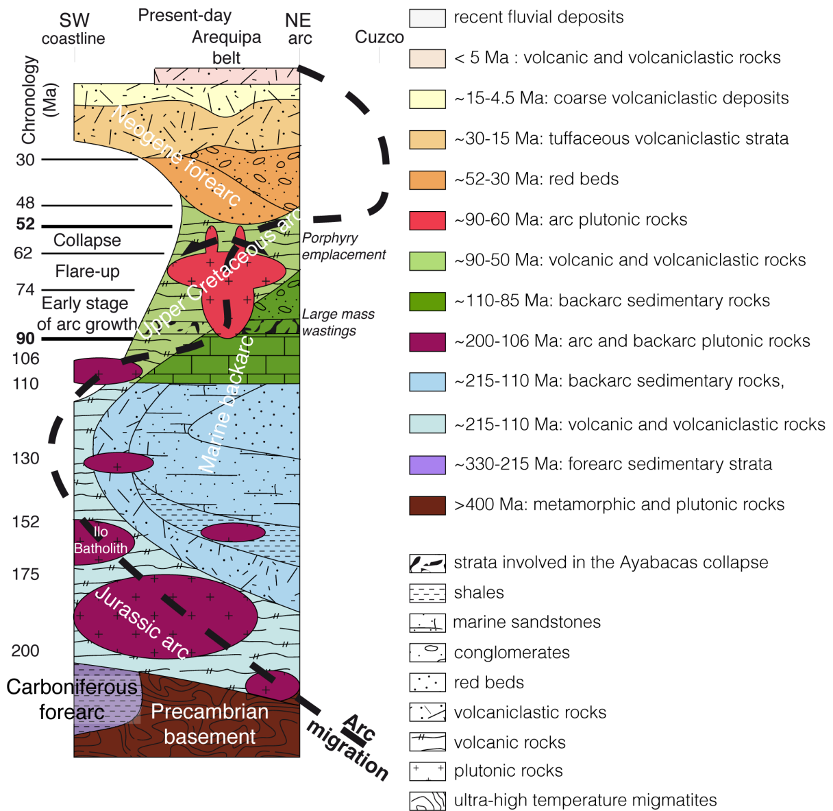
Figure C : Charte tectono-stratigraphique pour le sud du Pérou ; la verticale de droite correspond à la stratigraphie approximative sur la côte actuelle, celle de gauche à la stratigraphie supposée présente sous l'arc volcanique (telle qu'exposée dans la région de Huambo). Noter la migration de l'arc au cours du temps (ligne pointillée noire). Les tons clairs correspondent aux dépôts d'arc, les plus foncés à ceux d'arrière-arc.
