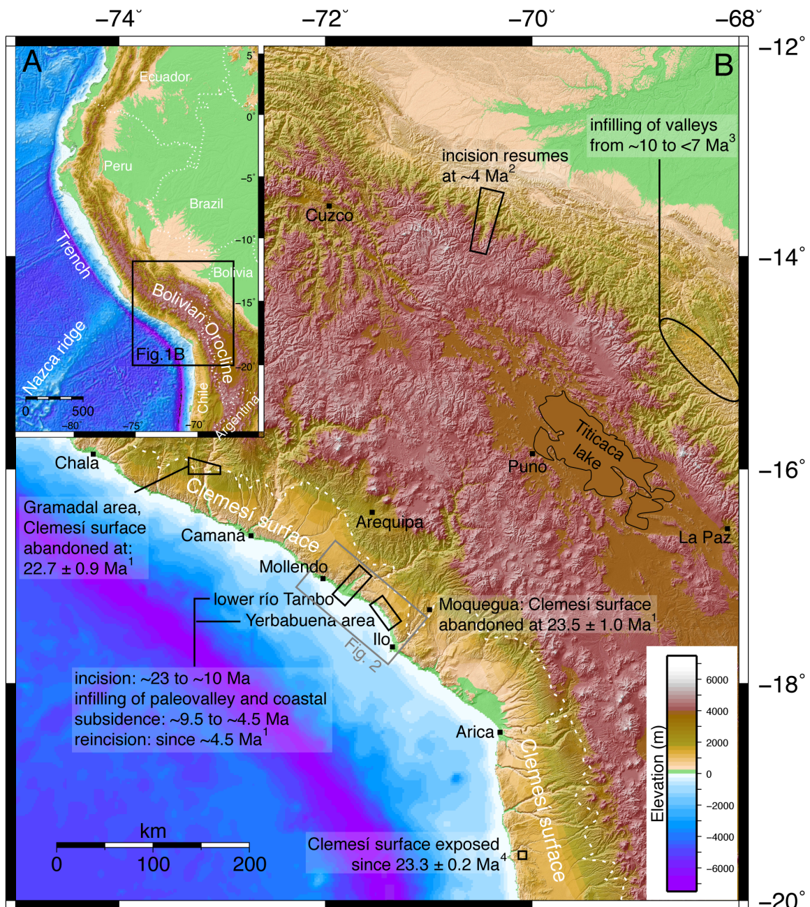
Figure I: Position et chronologie des différents évènements concernant le soulèvement des surfaces andines. La ligne pointillée blanche marque approximativement la limite NE de la surface Clemesi. Références : 1 : cette étude ; 2 : Lease & Ehlers (2013); 3 : Mosolf et al. (2011); 4 : Dunai et al. (2005).
