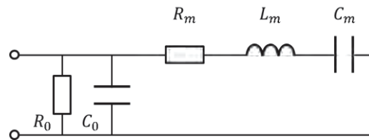
Figure 34 - Schéma électrique équivalent d'un transformateur piézoélectrique fonctionnant au voisinage de la résonance vu des bornes
