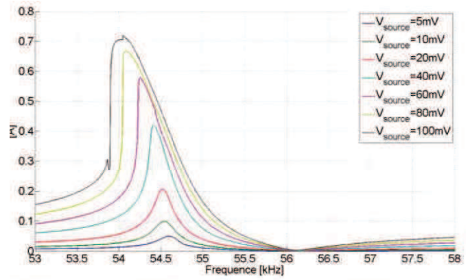
(b) Module de l'admittance – fréquence décroissante
