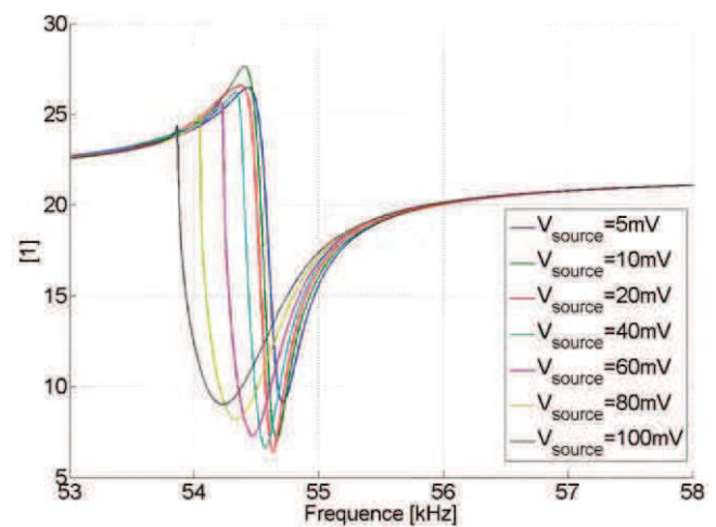
(f) Gain en tension – fréquence décroissante
