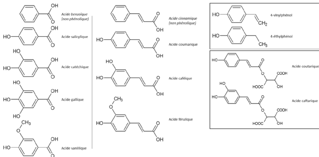
Figure 1 : Structures chimiques des principaux acides phénols du vin. A gauche les dérivés de l'acide benzoïque ; au centre, les dérivés de l'acide cinnamique ; à droite les phénols volatils et les esters de l'acide tartrique. (Roland, 2010; Navarre and Langlade, 2010; Ribéreau-Gayon et al. , 2012a)
