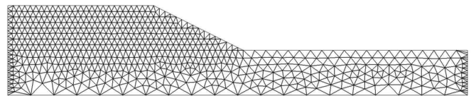
(d) Mesh 4 (25cm)
