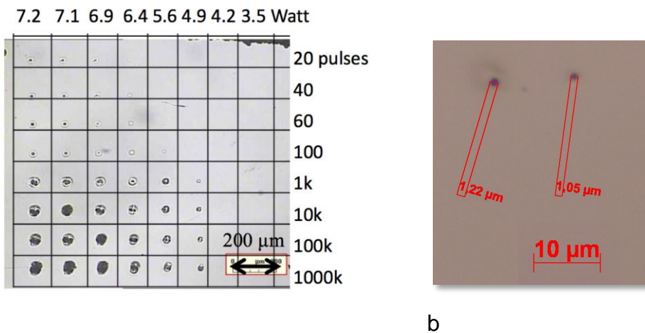
Figure 6. (a) Vue au microscope de gravures obtenues en sortie de la fibre optique en silice de 200 \mu\text{m} de cœur fonction de la puissance injectée et du nombre d'impulsions. (b) Vue des plus petites gravures réalisées avec la fibre en silice de 100 \mu\text{m} de cœur (35 impulsions, 7,2 W).
