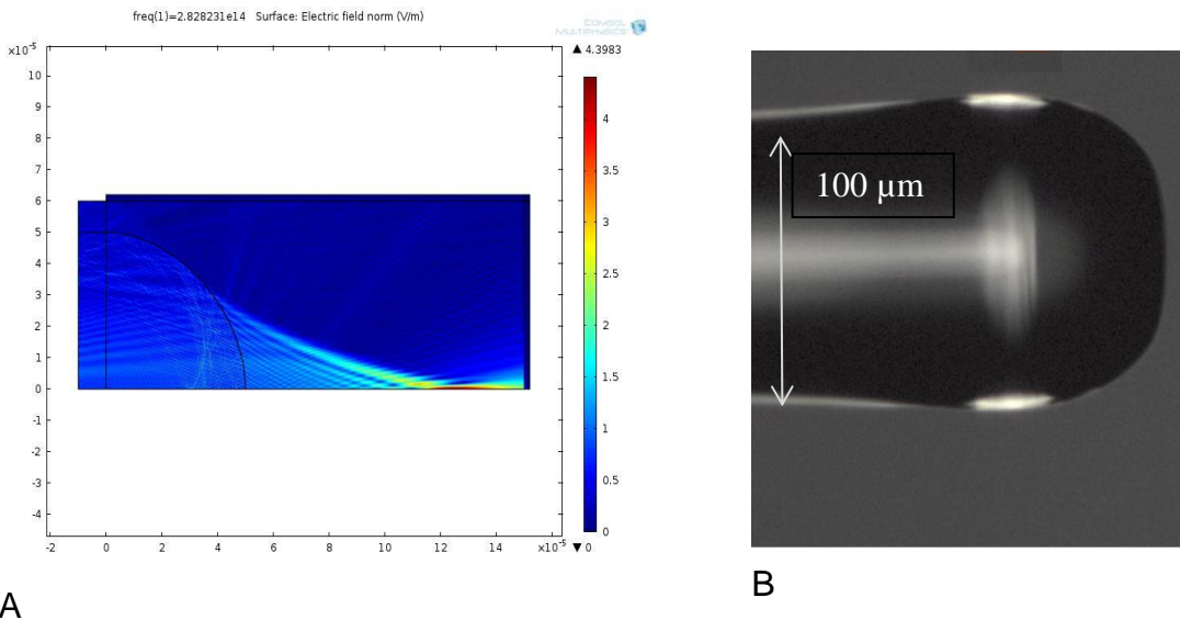
Figure 5. (a) Champ électrique en sortie d'un guide d'onde diélectrique planaire de 100 \mu\text{m} de cœur avec son embout sphérique. L'axe des x est un axe de symétrie. (b) Vue au microscope de la fibre correspondante réalisée pour effectuer les gravures.
