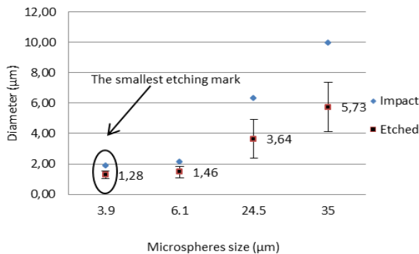
Figure 3 : Diamètre des gravures obtenues sur silicium en fonction du diamètre des billes de verres utilisées. Fluence incidente 0,7 \text{ J/cm}^2 . « Etched » : diamètre de la gravure centrale. « Impact » : taille globale de l'impact.
