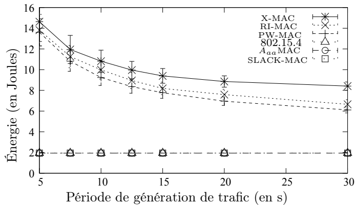
Figure 4.12 – Énergie moyenne consommée par heure par nœud en fonction de la période de génération de trafic, avec un taux d’activité fixe de 1 % pour IEEE 802.15.4, A_{aa} -MAC et SLACK-MAC et, avec un taux d’activité variable pour X-MAC, RI-MAC et PW-MAC.
