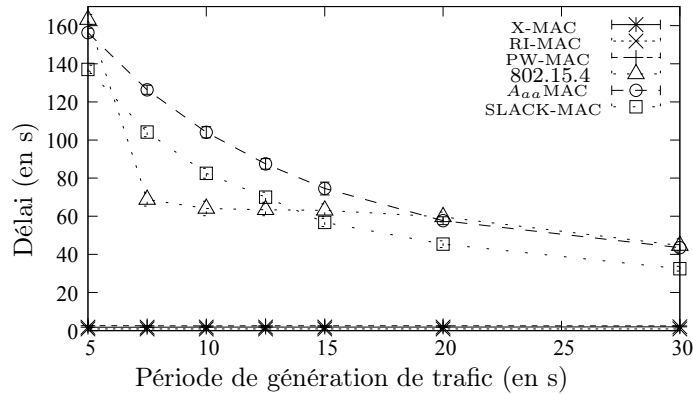
Figure 4.11 – Délai moyen de livraison des trames de données en fonction de leur période de génération, avec un taux d’activité fixe de 1 % pour IEEE 802.15.4, A_{aa} -MAC et SLACK-MAC, et avec un taux d’activité variable pour X-MAC, RI-MAC et PW-MAC.
