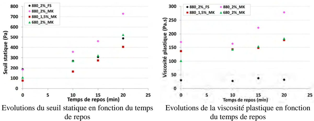
Figure 3 - 8 : Evolutions du seuil statique et de viscosité plastique en fonction du temps de repos
