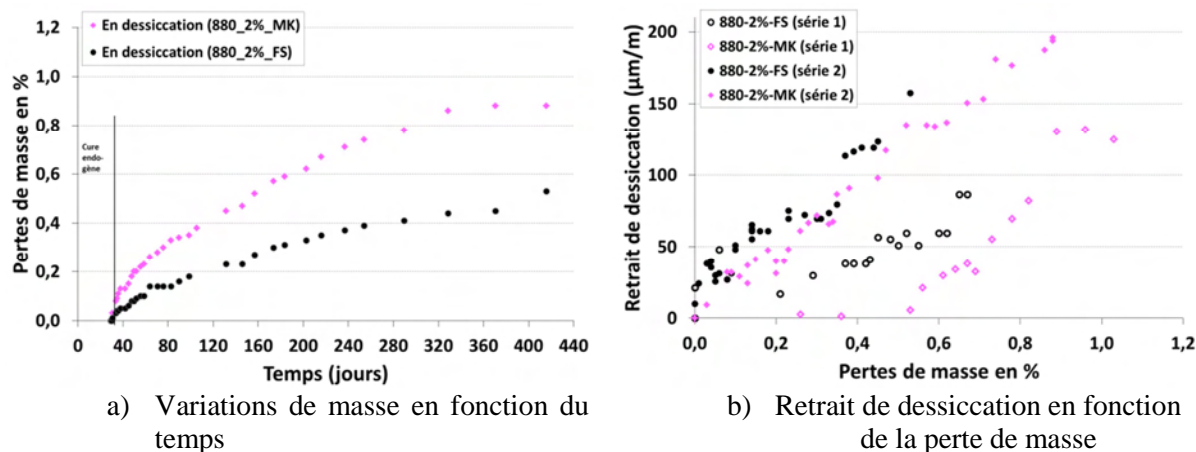
Figure 4 – 23 : a) Perte de masse en fonction du temps ; b) Retrait de dessiccation en fonction de la perte de masse des BFUP 880_2%_FS et 880_2%_MK
