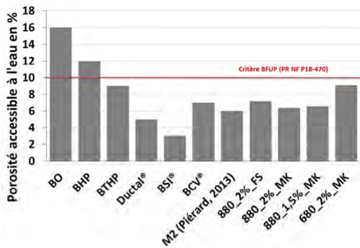
Figure 5 – 7 : Porosité accessible à l'eau de différents bétons
