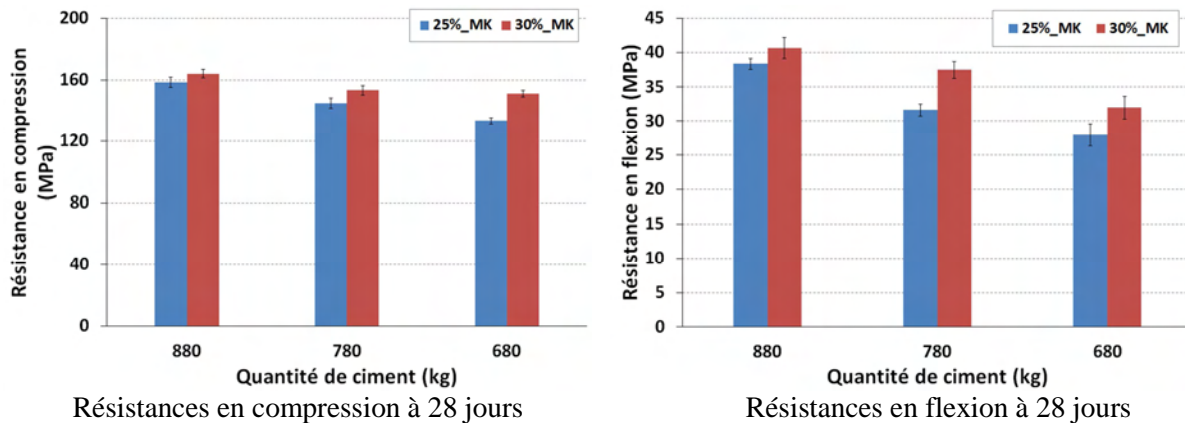
Figure 2 – 8 : Comparaison de résistances mécaniques à 28 jours des différentes formulations testées en fonction du dosage en ciment et du taux d'incorporation du métakaolin
