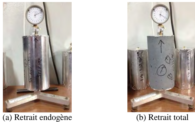
Figure 4 - 9: Dispositif de mesure de retrait
