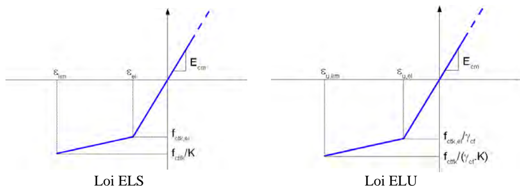
Figure 1 - 25 : Loi pour les BFUP de classe T3 (obtenue directement en \sigma(\epsilon) ) selon (PR NF P18-710)
