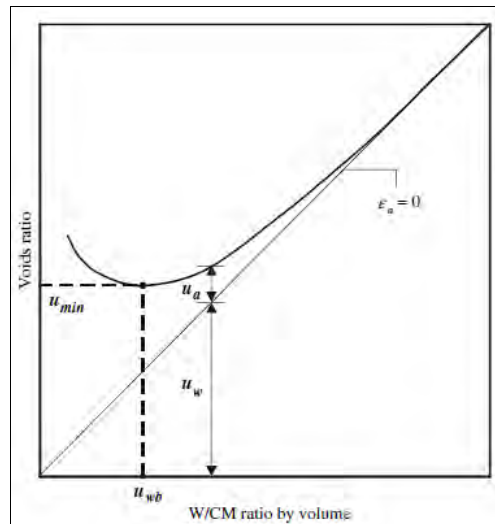
Figure 2 – 6 : Représentation du ratio des vides (voies ratio) en fonction du rapport volumique Eau/Poudre (W/CM ratio by volume) pour un taux de substitution donné de A/C (Kwan et al., 2012)
