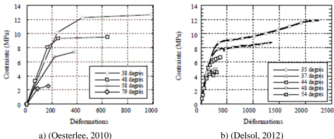
Figure 1 - 13 : Comportement en traction directe pour différentes orientations de fibres : (a) : selon (Oosterlee, 2010); (b) : selon (Delsol, 2012)
