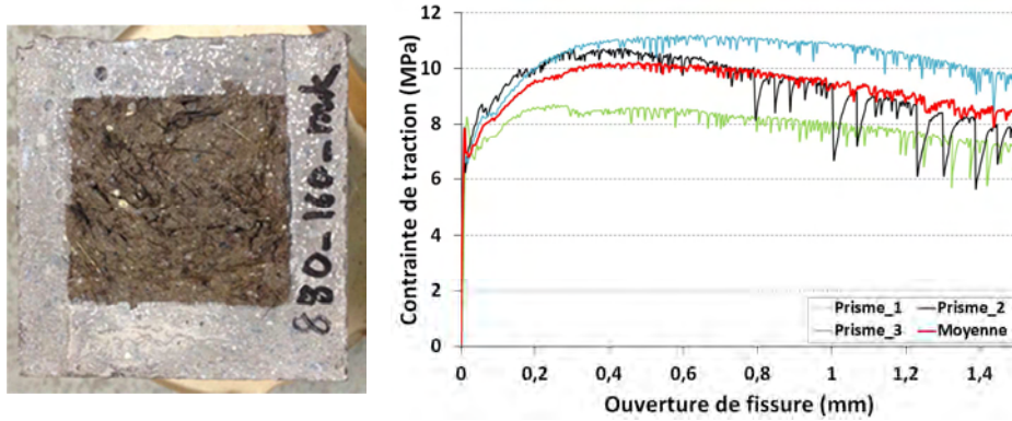
Figure 4 – 18 : Aspect de l'échantillon après rupture et courbes contrainte de traction – ouverture de fissure pour le béton 880-2%-MK obtenues lors d'essais de traction directe
