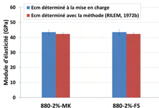
Figure 4 – 24 : Comparaison des modules d'élasticité des deux BFUP 880-2%-FS et 880-2%-MK déterminés à la mise en charge et par la méthode (RILEM, 1972)
