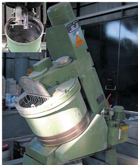
Figure 1 - 4 : Malaxeur EIRICH R08W
