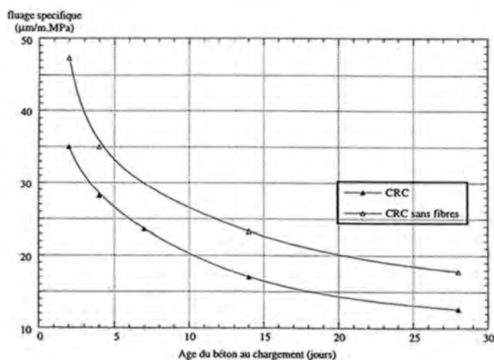
Figure 1 - 20: Influence de la présence de fibres sur le fluage propre spécifique en compression du CRC à différents âges de chargement (Loukili, 1996)
