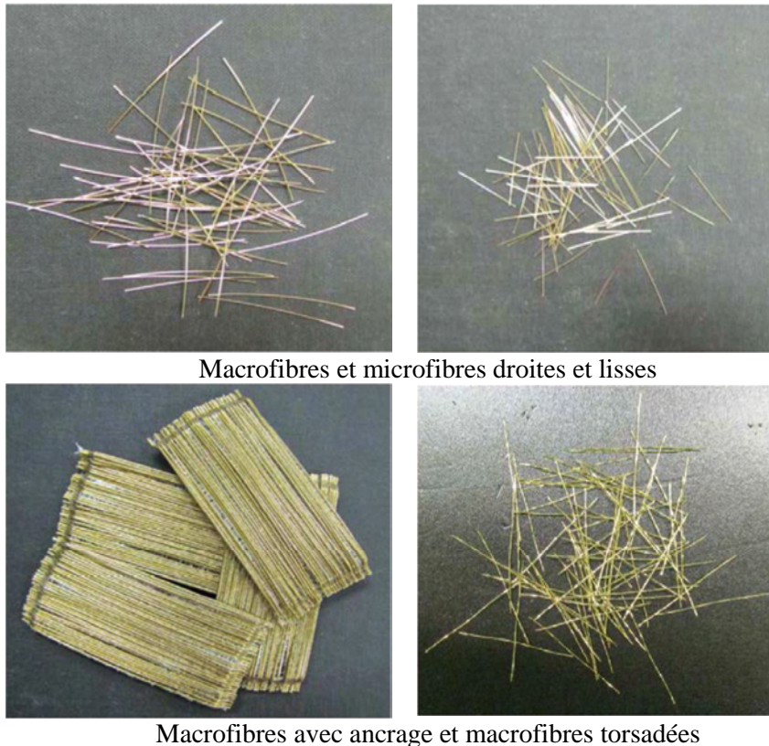
Figure 1 - 1: Photographies illustrant les différents types des fibres métalliques pouvant être incorporées dans les BFUP
