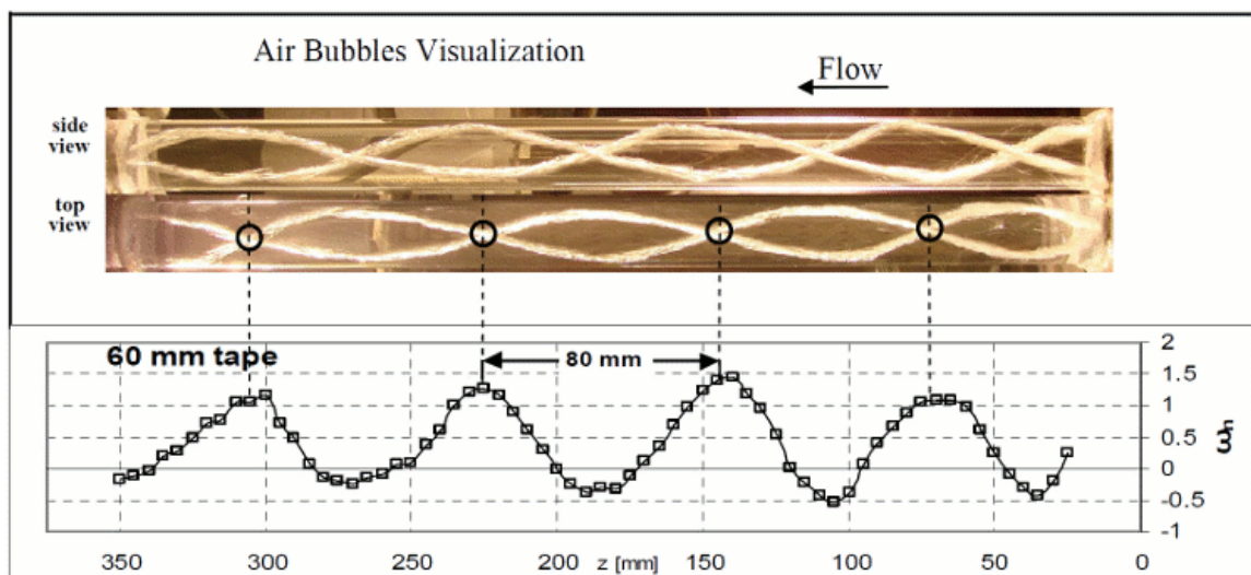
FIGURE 1.11 – Comparaison entre l’angle de rotation normalisé mesuré au centre de la conduite par méthode LDV et les visualisations par injection de bulles d’air, pour un écoulement en aval d’une ailette torsadée sur 180^\circ (swirler court), illustration de [12].
