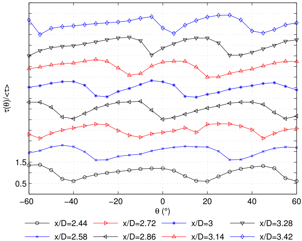
FIGURE 4.17 – Distribution circouférentielle du frottement adimensionné \frac{\tau}{\langle\tau\rangle} sur un intervalle de 120^\circ discrétisé par pas de 5^\circ pour 8 sondes successives espacées de 5 mm à Re_D = 2000 (référence arbitraire).
