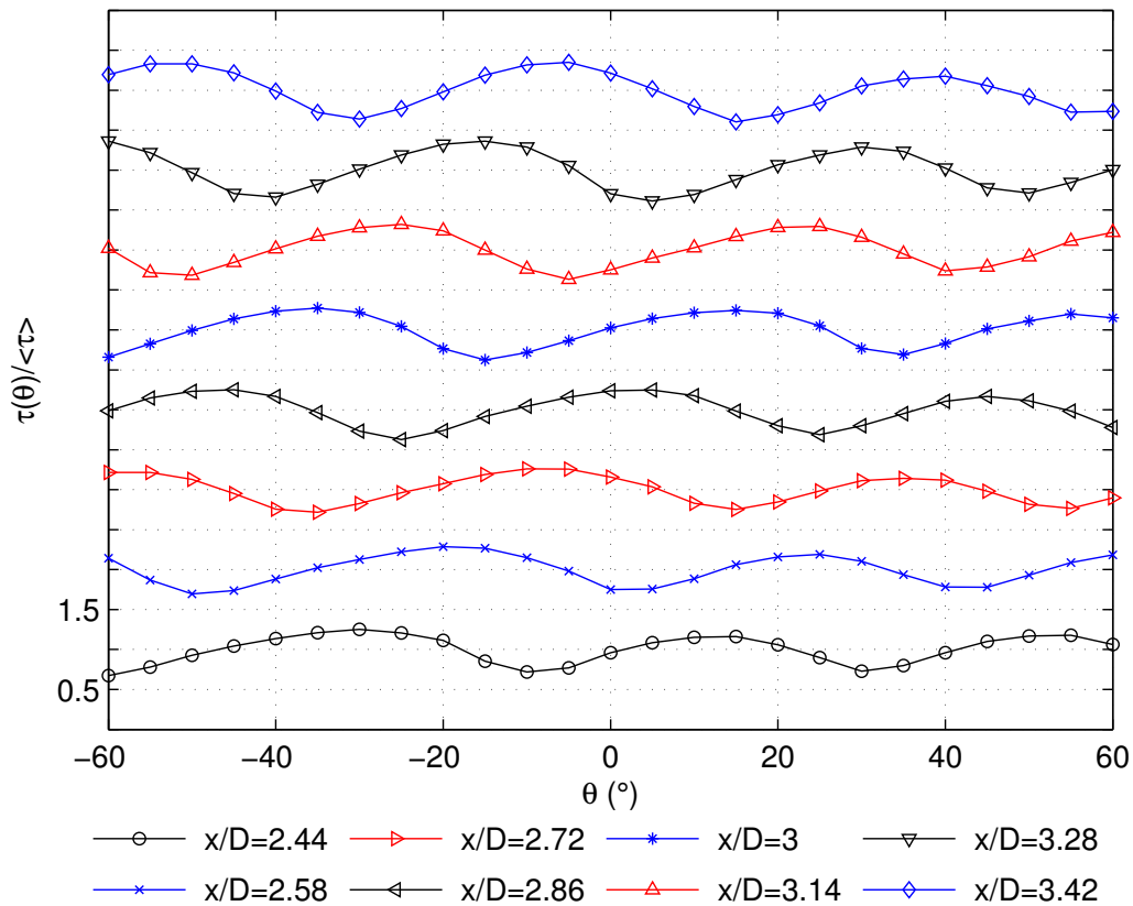
FIGURE 4.16 – Distribution circumférentielle du frottement adimensionné \frac{\tau}{\langle\tau\rangle} sur un intervalle de 120^\circ discrétisé par pas de 5^\circ pour 8 sondes successives espacées de 5 mm à Re_D = 1000 (référence arbitraire).
