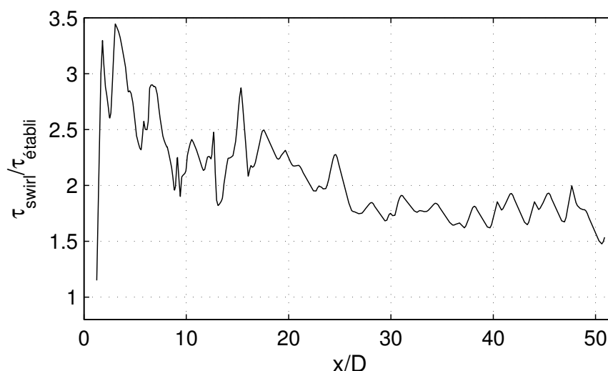
FIGURE 4.23 – Distribution axiale du rapport de frottement \frac{\tau_{\text{swirl}}}{\tau_{\text{\u00e9tabli}}} en fonction de x/D pour un \u00e9coulement \u00e0 Re_D = 2000 .
