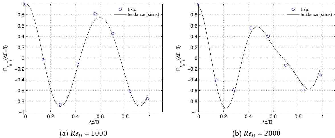
FIGURE 4.20 – Coefficients d'intercorrélations sur les valeurs moyennes du frottement à décalage angulaire nul.
