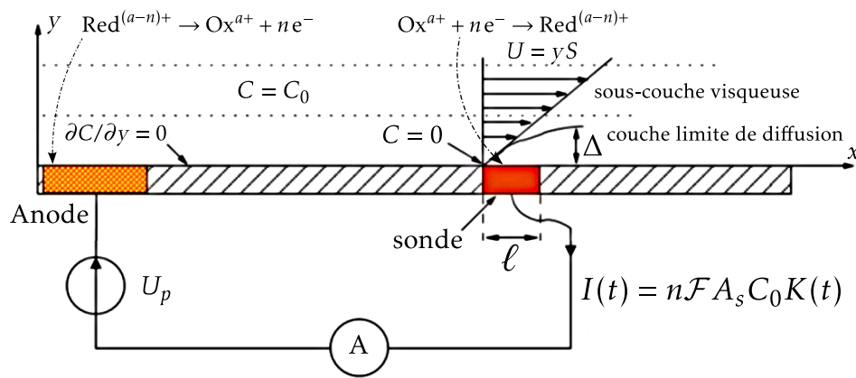
FIGURE 2.13 – Schéma de principe de la méthode électrochimique.
