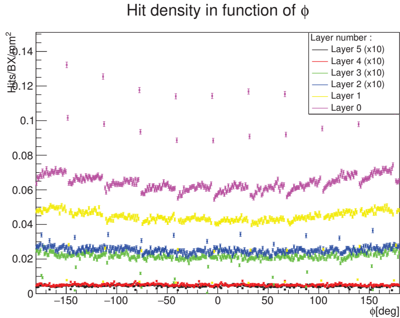
FIGURE 6.4 – Densité d'impact de bruit de fond en Impacts/BX/mm^2 en fonction de l'angle cylindrique \phi et de la couche du détecteur de vertex. La densité d'impacts est moyennée sur 1325 croisements de faisceaux.
