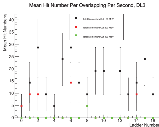
FIGURE 6.23 – Statistique estimée pour les extrémités des échelles de la double couche 3 en fonction du numéro d'échelle, pour 3 valeurs d'impulsion minimales. (100, 200 et 400 \text{ MeV}/c ).
