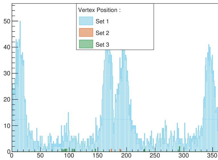
FIGURE C.31 – Angle local \phi associé à chaque impact de bruit de fond de la couche 5 pour les impacts associés à des impulsions supérieures à 100 \text{ MeV}/c .
