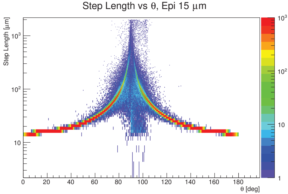
FIGURE 6.25 – Longueurs traversées par une particule incidente dans la couche épitaxiée d'un capteur en fonction de l'angle d'incidence \theta . Une couche épitaxiée de 15 \mu m est utilisée.
