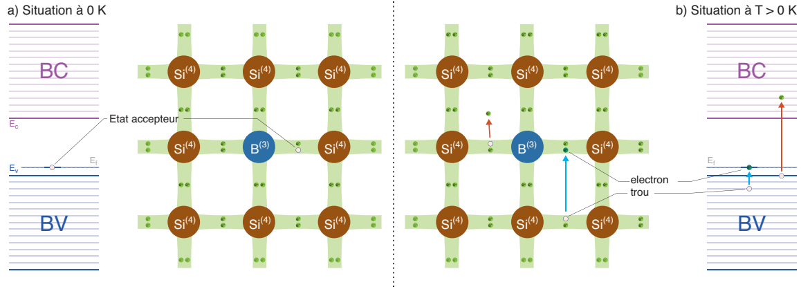
FIGURE 3.5 – Représentation schématique des liaisons électroniques pour un semi-conducteur dopé de type P et positions d'électrons dans les bandes (a) à T = 0 K et (b) à T > 0 K. Le bore de valence trois a un électron en moins par rapport à l'atome de silicium qu'il remplace dans le réseau. Les quatre liaisons covalentes ne sont pas pleinement satisfaites, et la présence de l'atome de bore introduit de fait un état vide faiblement lié qu'on appelle un état accepteur (d'électron) situé proche de la bande de valence.
