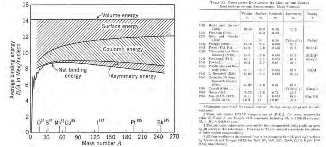
FIGURE 1.2 – Évolution des l'énergie de liaison par nucléon B/A en fonction de la masse A en regard des contributions des différents termes de la formule de Bethe-Weizsäcker [Eva55].
