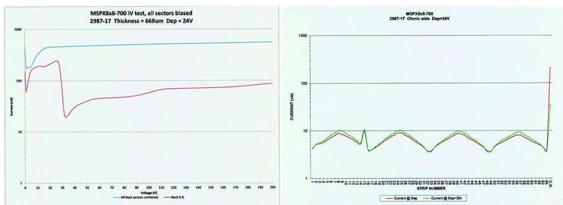
FIGURE 8.12 – Graphe représentant les courants du détecteur 3D 17 à gauche en fonction de la tension de polarisation et à droite pixel par pixel, à la tension de déplétion et à Vd+30V.
