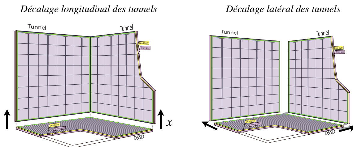
FIGURE 5.16 – Décalage longitudinal (à gauche) et latéral (à droite) des Tunnel par rapport au DSSD.
