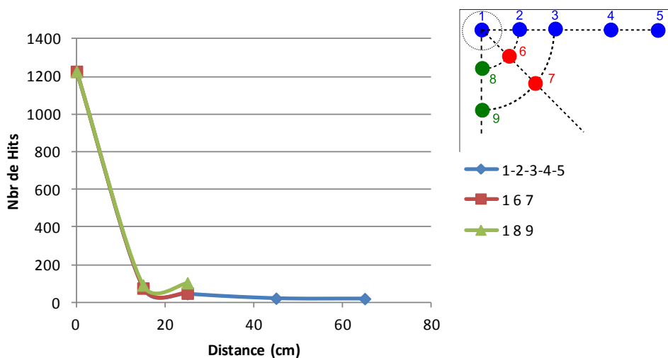
Figure 3-48 Graphique présentant le nombre de hits enregistrés par les capteurs en fonction de la distance et de l'orientation
