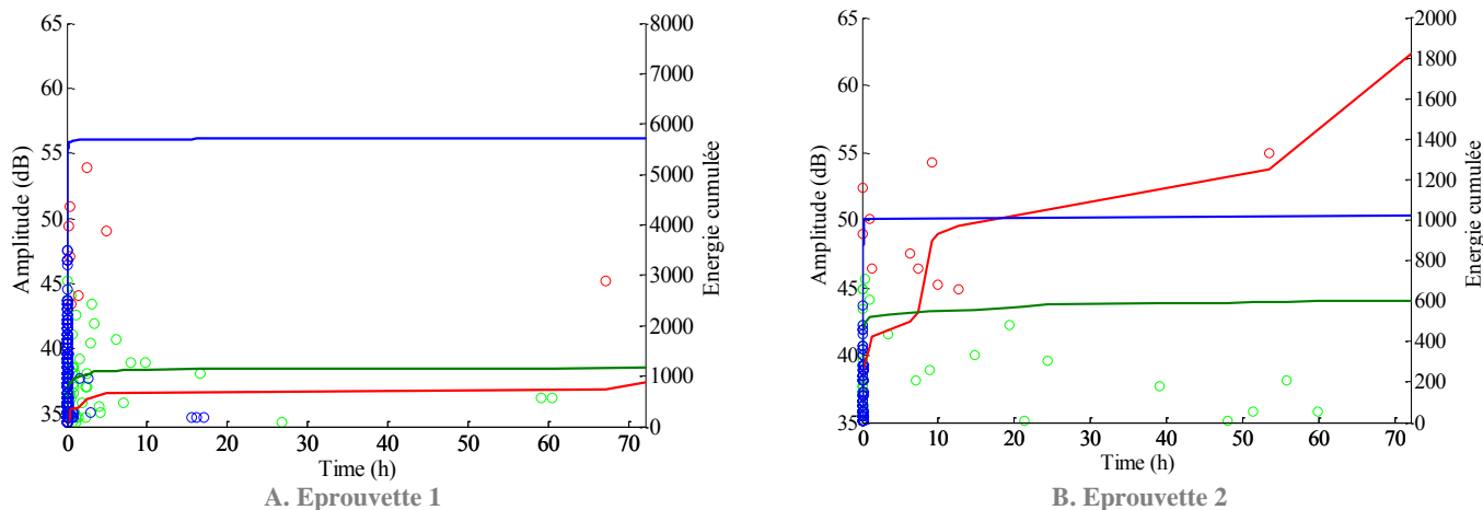
Figure 3-25 Energie cumulée en fonction du temps pour les différentes classes
