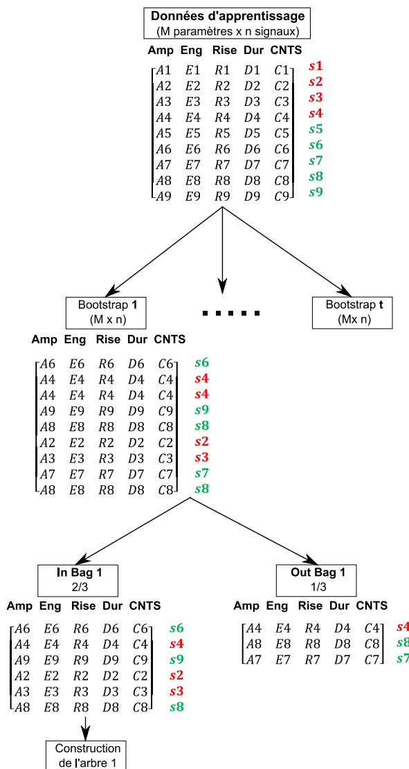
Figure 3-7 Préparation des données et obtention des données « In Bag ».
