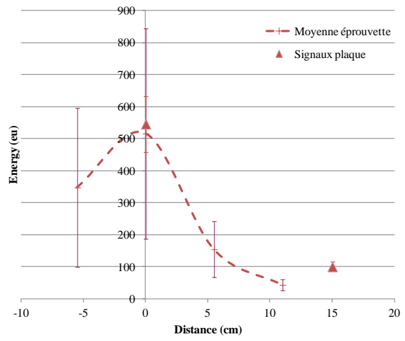
D. Evolution de l'énergie en fonction de la distance du capteur pour les signaux de la classe rupture
