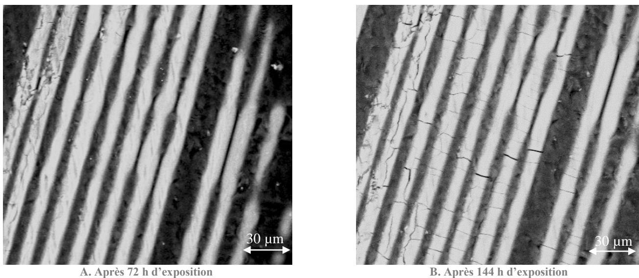
Figure 3-27 Images MEB de l'éprouvette n°1 après 72 h et 144 h d'exposition
