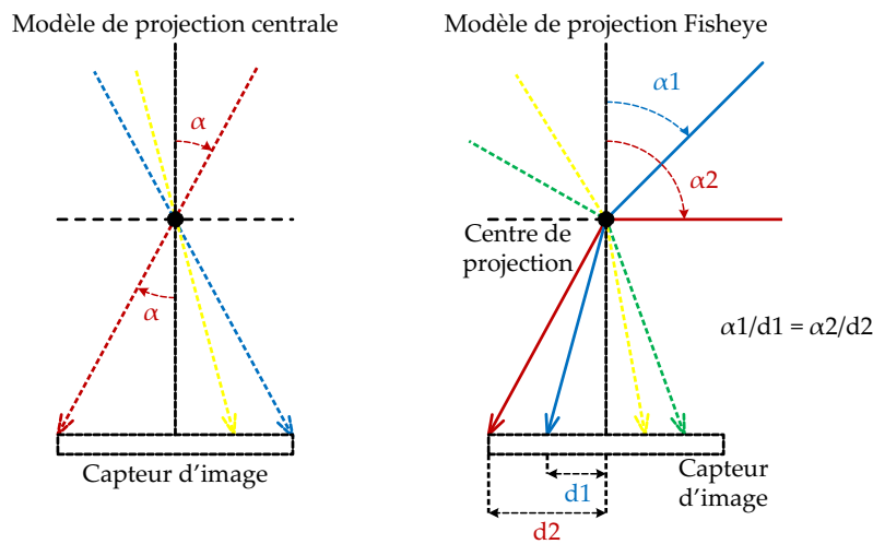
FIGURE 2.4: Comparaison de la projection centrale du modèle sténopé à gauche, avec la projection Fisheye à droite.
