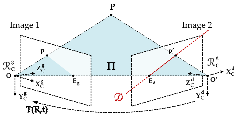
FIGURE 4.7: Géométrie épipolaire classique. Un point P est projeté sur deux images et donne naissance aux points m(u, v) et m'(u', v') .
