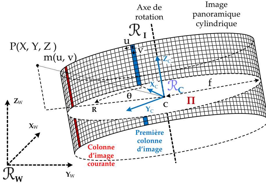
FIGURE 4.2: Modèle géométrique proposé dans les travaux de L. Smadja et al. en 2004 "Cylindrical Sensor Calibration using Lines"
