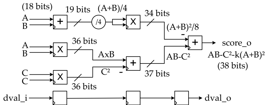
FIGURE 3.23: Illustration de l'étape finale du calcul des scores de Harris et Stephens. Trois cycles d'horloge sont nécessaires à la réalisation de ce calcul.
