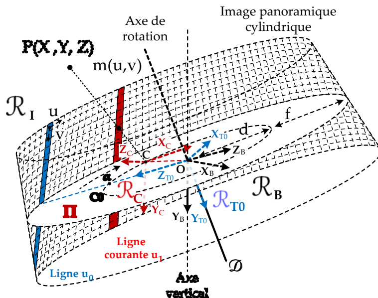
FIGURE 4.5: Modèle général d'un système à caméra linéaire rotatif. On constatera que l'image n'est pas tout à fait un cylindre, cela est due à la modélisation des trois angles (\phi, \theta, \psi) de l'erreur d'orientation du capteur. Cela pose le problème de la résolution non-homogène.
