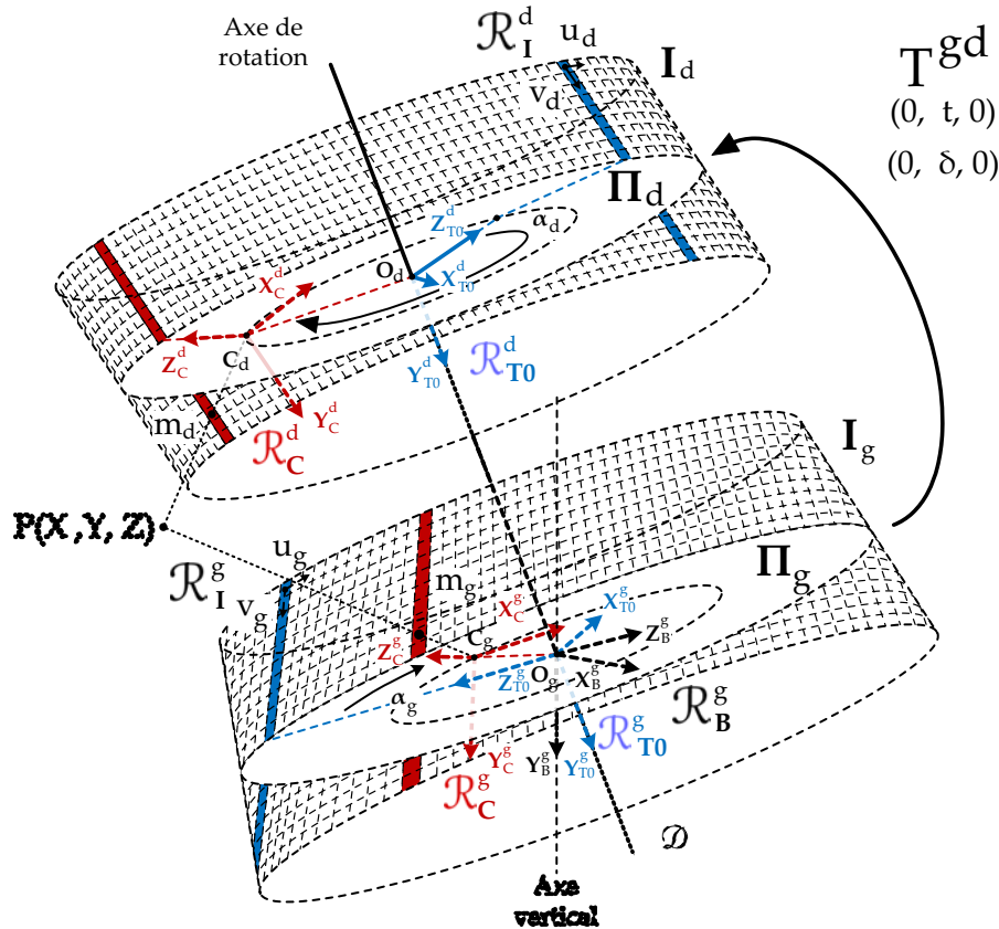
FIGURE 4.11: Modèle général d'un stéréoscopique à caméras linéaires rotatives. On constatera que les deux images ne sont pas tout à fait des cylindres, cela est dû à la modélisation des angles (\phi_d, \theta_d, \psi_d) et (\phi_g, \theta_g, \psi_g) de l'erreur d'orientation des capteurs.
