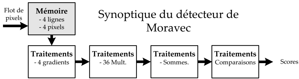
FIGURE 3.13: Synoptique de l'organisation en Pipe-Line du détecteur de Moravec
