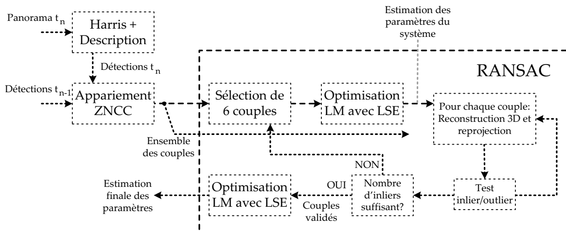
FIGURE 5.5: Synoptique de notre algorithme de localisation.
