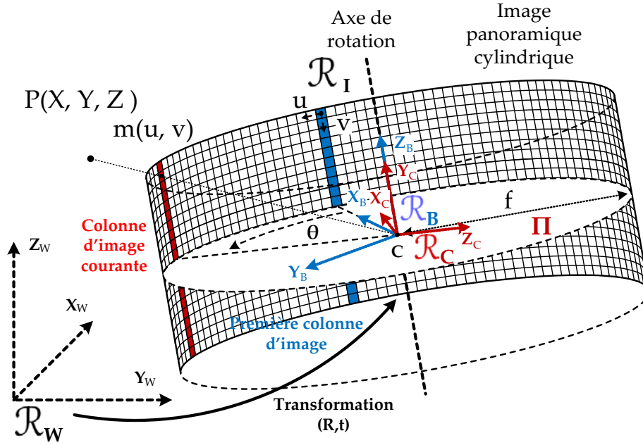
FIGURE 4.3: Modèle géométrique proposé dans les travaux de Parian et al. en 2004 "A Refined Sensor Model For Panoramic Cameras".
