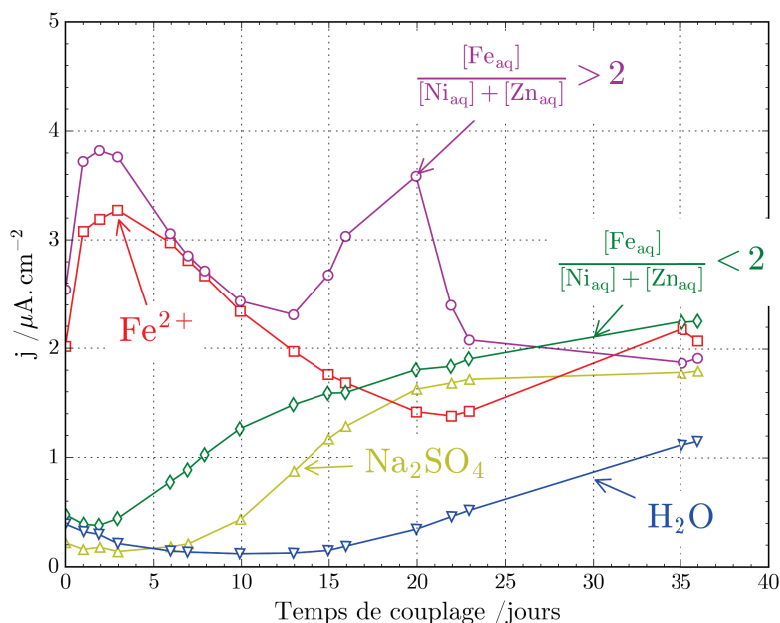
FIGURE 4.2 – Evolution dans le temps des densités de courant de couplage pour les cinq électrolytes choisis.
