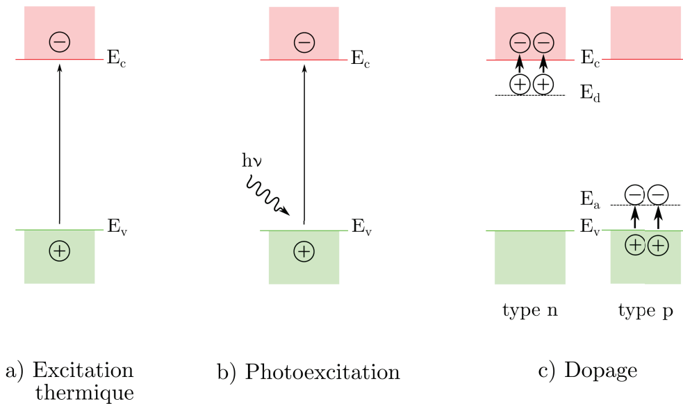
FIGURE 1.31 – Représentation schématique des mécanismes de génération des porteurs de charge dans des semiconducteurs ou des isolants (d'après FINKLEA [75]) : a) excitation thermique, b) photoexcitation, c) dopage.
