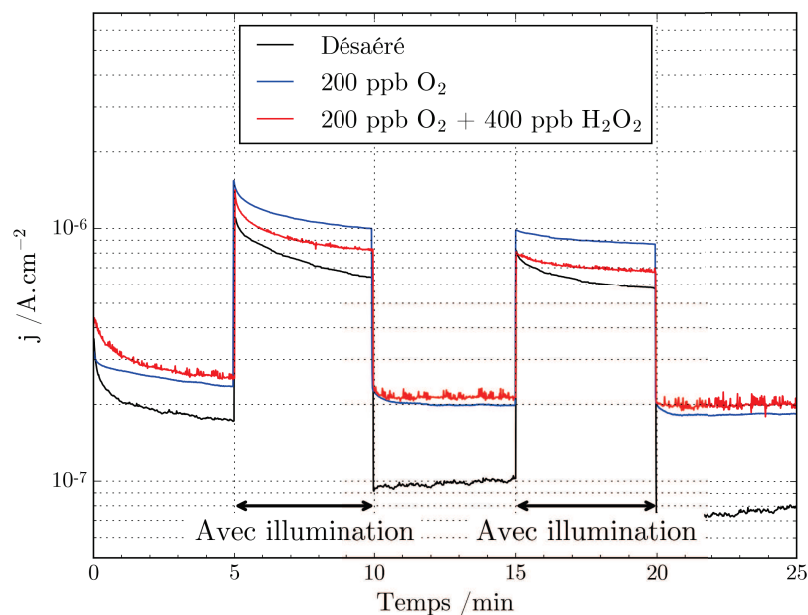
FIGURE 4.19 – Evolution de la densité de courant de couplage avec et sans illumination UV–Visible pour les trois électrolytes considérés. "Avec illumination" indique les périodes où l'échantillon est illuminé de manière continue avec la lampe Hg.
