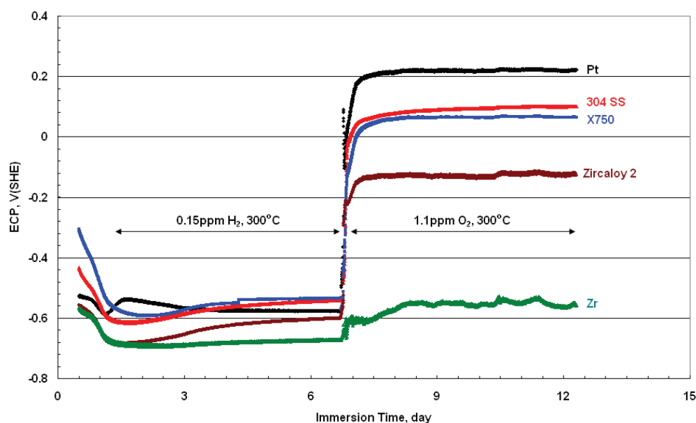
FIGURE 1.27 – Evolution des potentiels électrochimiques de l'alliage Zircaloy-2, de l'acier inoxydable 304, de l'alliage de nickel X750 et du Pt dans l'eau à 300 \text{ }^\circ\text{C} contenant 0.15 ppm de H_2 ou 1.1 ppm d' O_2 [57].
