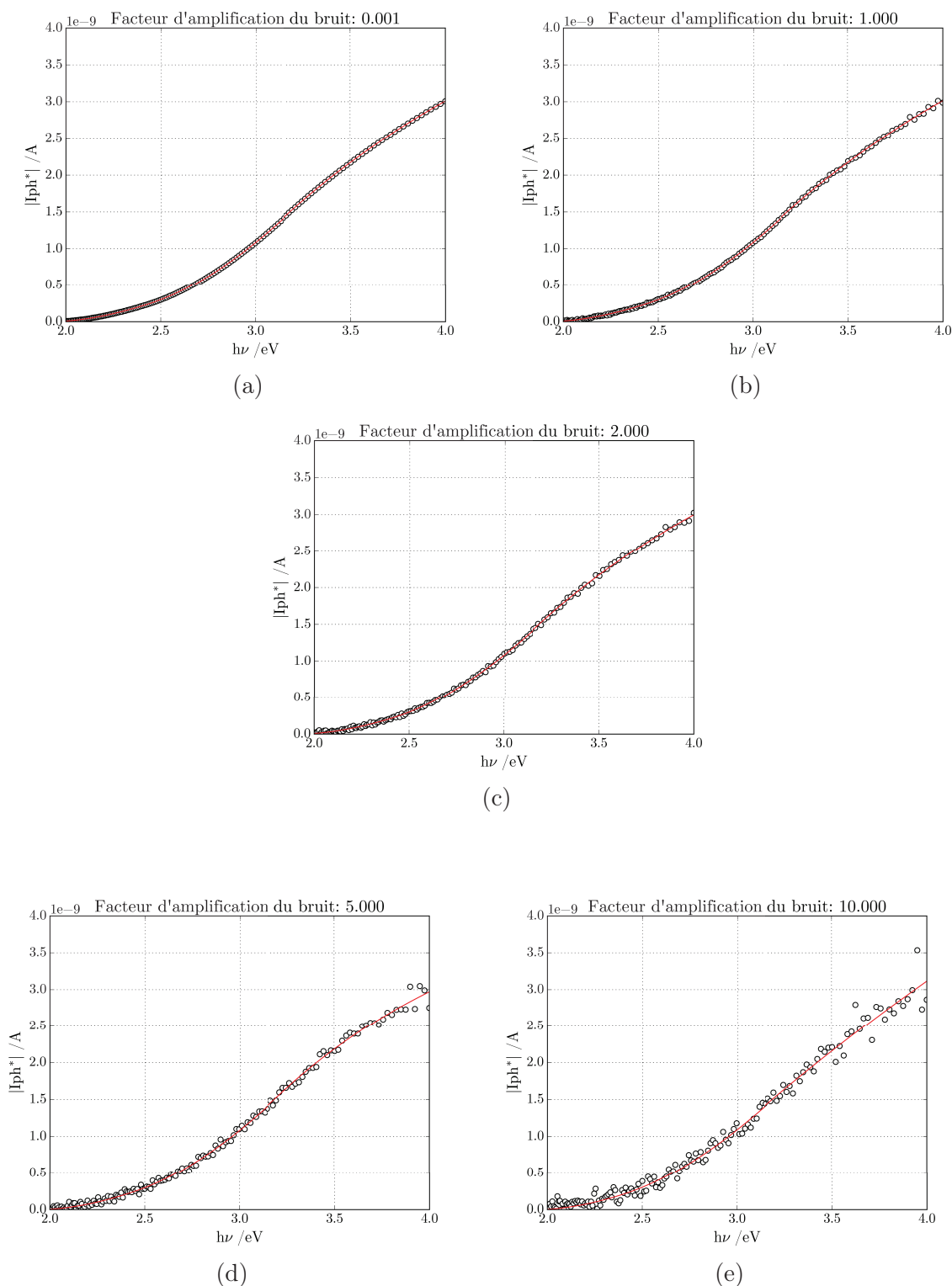
FIGURE 3.8 – Photocaractéristiques en énergie générées avec différents facteurs d'amplification du bruit ( f_a ) : a) 0.001, b) 1, c) 2, d) 5, e) 10.
