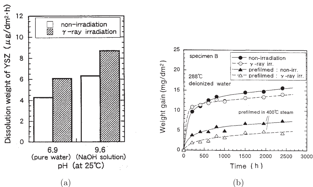
FIGURE 1.13 – Effet de l'irradiation \gamma : a) perte de masse de la zircone massive stabilisée à l'yttrium dans l'eau à 25 °C sous irradiation, b) prise de masse de alliage Zircaloy-2 dans de l'eau pure à 288 °C sous irradiation \gamma [43].
