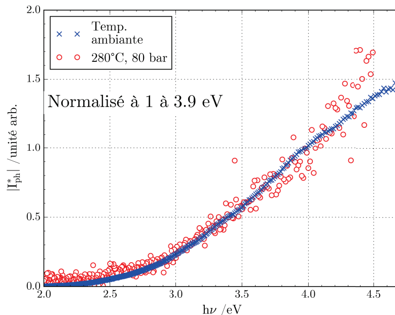
FIGURE 4.30 – Spectres en énergie de photocourants obtenus sur l’alliage de nickel X750 oxydé (280 °C et 80 bar en eau ultra pure) avec le dispositif expérimental HTP développé dans ce travail. Les photocourants ont été normalisés à 1 à 3.9 eV.
