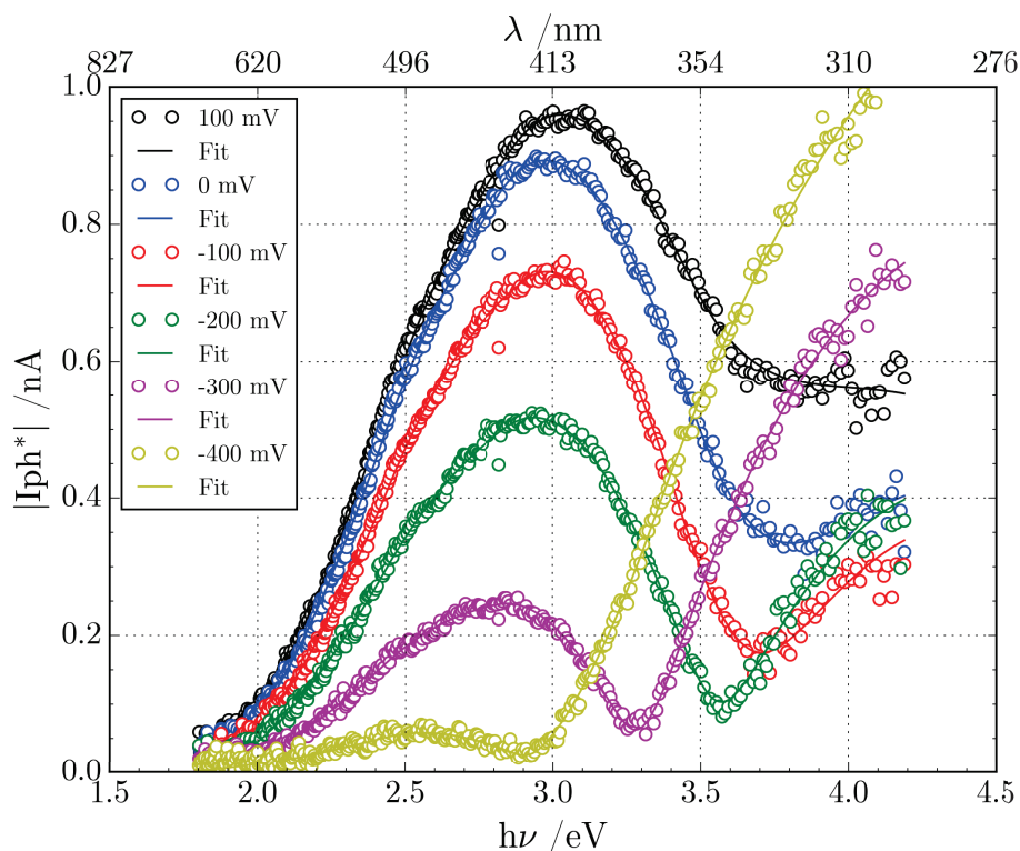
FIGURE 3.7 – Photocaractéristiques en énergie ( I_{\text{ph}}^* ) mesurées à plusieurs potentiels sur l'alliage A600 oxydé thermiquement (d'après PETIT et al. [1]).
