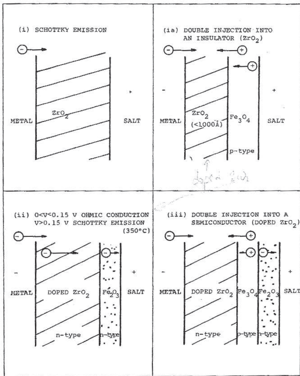
FIGURE 1.8 – Modèles de couche d'oxyde sur les intermétalliques de l'alliage Zircaloy-2 [28].
