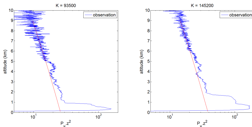
FIGURE 3.2 – Profils LiDAR réalisés sur Paris à l'issue des réglages avec deux systèmes fabriqués pour IAOS. Le profil atmosphérique US 1976 a été utilisé. La zone moléculaire utilisée pour le calcul de la constante système atténuée est situé entre 5.5km et 7km. La valeur réelle de la constante système (indiquée au dessus de chaque courbe) est alors obtenue en considérant une atténuation de 10% (mesurée en moyenne par le réseau AERONET sur Paris) par les aérosols sous la zone moléculaire. Le signal moléculaire est alors tracé (courbe rouge) en prenant en compte la valeur réelle de la constante système. Comme prévu il y a une absence de superposition entre la zone moléculaire du signal et le signal moléculaire théorique pur. Pour le profil de gauche, la valeur plus faible peut s'expliquer par une fonction de recouvrement particulièrement faible ou alors par la présence d'aérosols particulièrement absorbant au moment de l'observation. Pour le profil de droite, une transmission légèrement meilleure que celle indiquée dans le tableau 3.1 peut expliquer cette valeur légèrement supérieure. Quoiqu'il en soit ces deux exemples se situent dans le panel des valeurs attendues à \pm 10\% .
