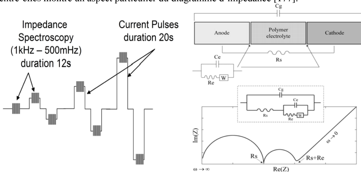
Figure. II. 24: Identification fréquentielle [178]
