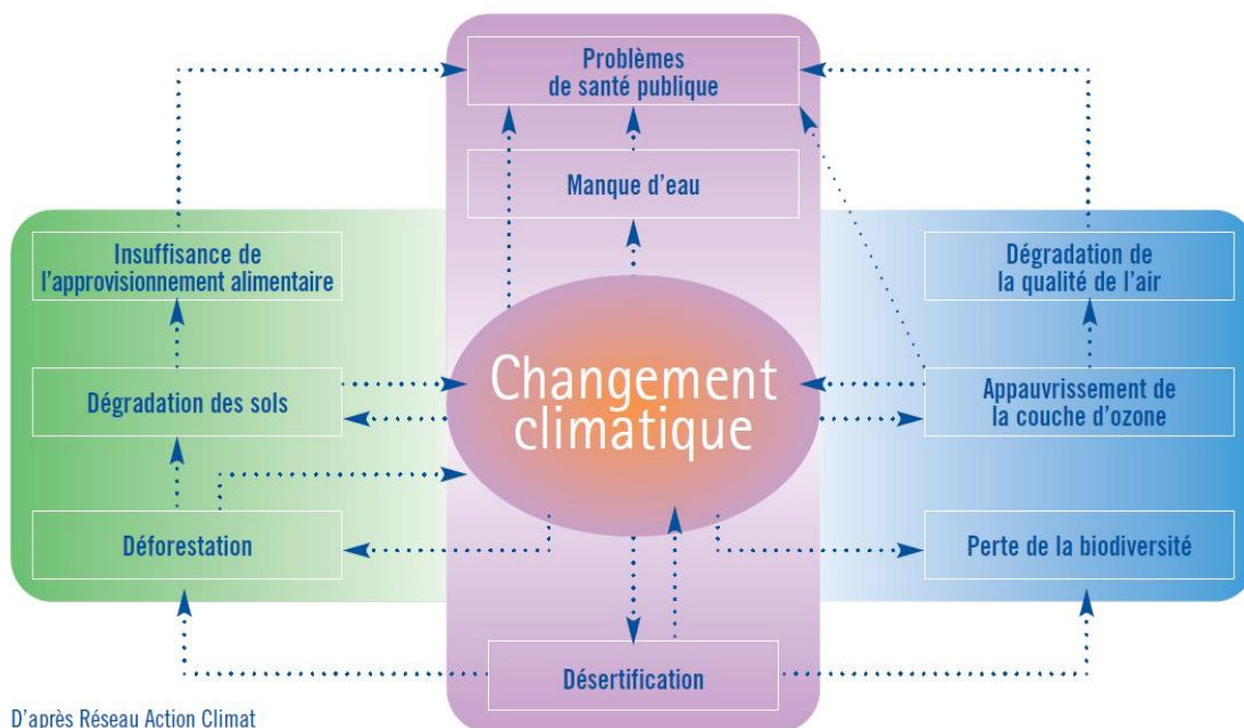
Figure. I. 3: Impacts environnementaux liés aux changements climatiques [16]
