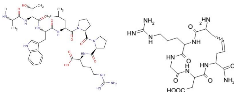
Figure 15 Le peptide ATWLPPR (gauche) et le RGD (droite)
