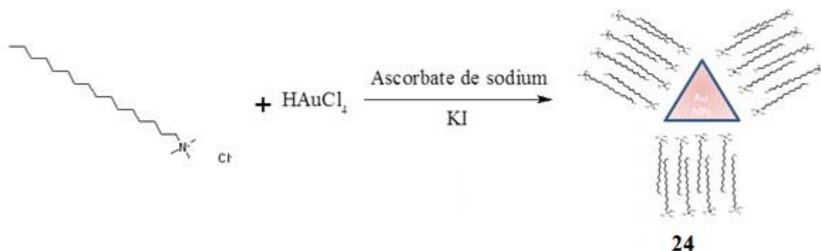
Figure 88 Synthèse d'AuNPs triangulaire (24) en présence de CTAC
