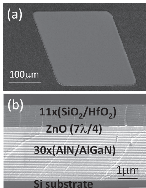
FIGURE 2.3 – Images de microscopie électronique à balayage de la cavité \text{ZnO} à mesas (a) Vue du dessus d'une mesa de forme "diamant" sans cracks visibles à la surface (b) Coupe complète de la microcavité avec indication de la composition des couches.
