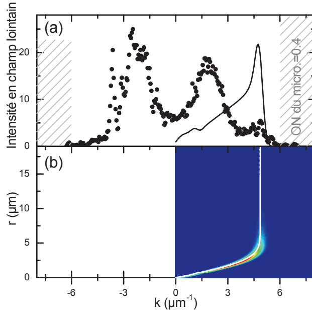
FIGURE 3.12 – (a) Profils expérimentaux en k_y du condensat en champ lointain (poinillés) au-dessus du seuil du laser à polaritons ( P = 1.7P_{th} , LPB1, T=300 K), et simulation GPE liée aux figures 3.11.c et d (trait plein). (b) Relation entre vecteur d’onde et rayon de propagation du condensat. L’intensité d’émission est en fausses couleurs.
