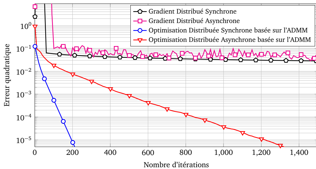
Figure IV.2 : Erreur quadratique en fonction du nombre d'itérations pour différents algorithmes d'optimisation distribuée.
