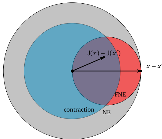
Figure IV.1 : Illustration de la ferme non-expansivité.
