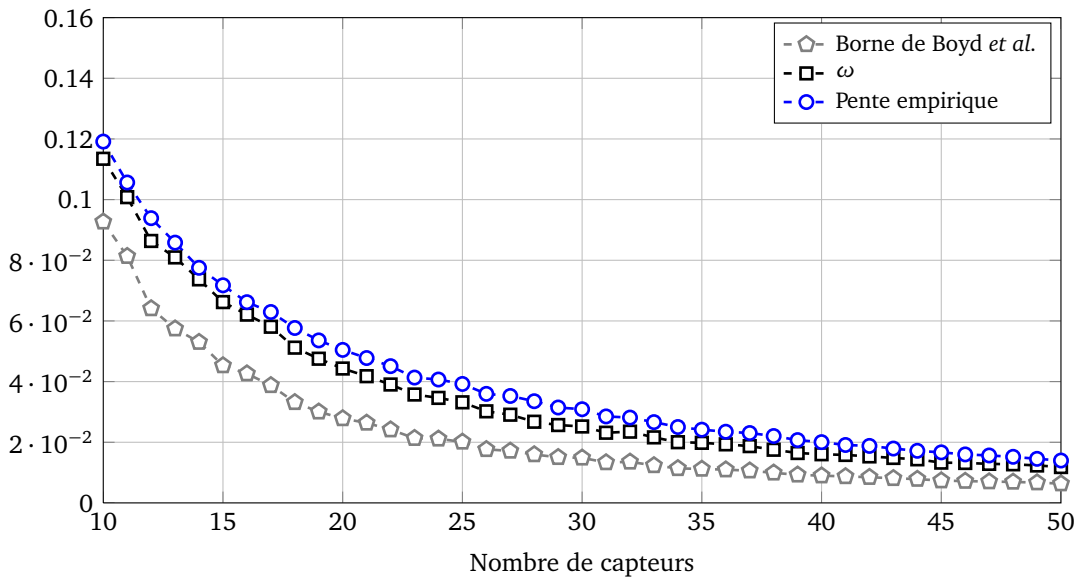
Figure III.3 : Pente empirique du logarithme de l'EQM du Random Gossip et bornes associées.
