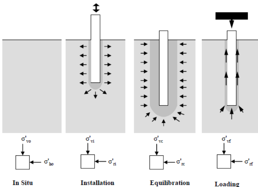
Figure I - 3 - Evolution de l'état des contraintes effectives autour du pieu en fonction du temps (Doherty and Gavin, 2011)
