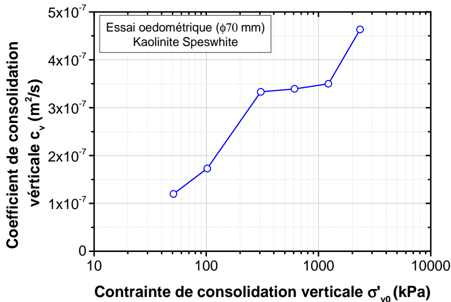
Figure II - 33 - Evolution du coefficient c_v ( m^2/s ) en fonction de la contraente de consolidation
