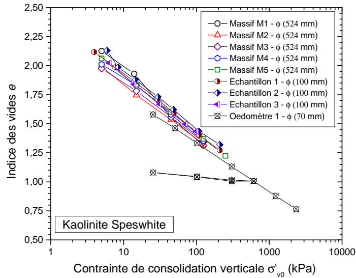
Figure II - 39 - Comparaison entre les massifs (φ 524 mm) et les éprouvettes (φ 100 mm)
