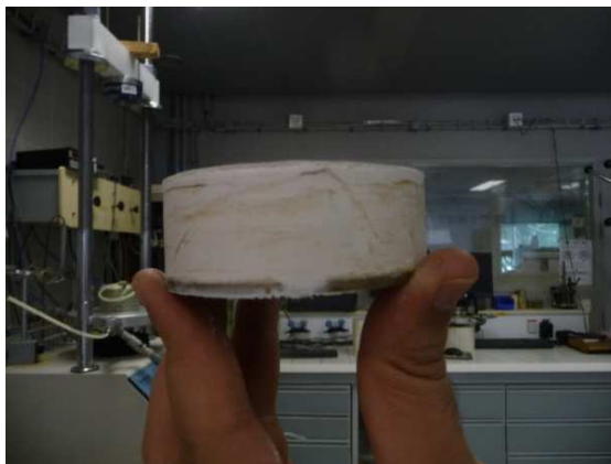
Figure II - 35 - Vue de l'éprouvette après l'essai de compressibilité œdométrique
