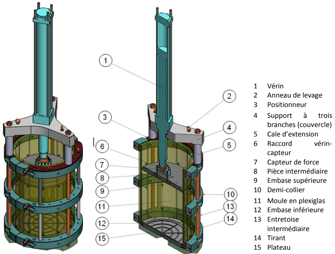
Figure II - 15 – Dessin 3D représentant le dispositif de reconstitution des massifs d'argile par consolidation (consolidomètre)
