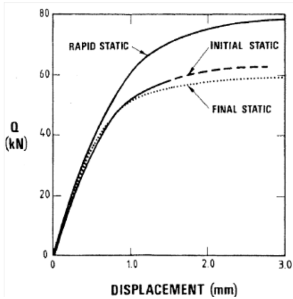
Figure I - 15 - Effet de la vitesse de chargement sur la capacité portante des pieux in situ installés dans l'argile de Haga (Karlsruud et al., 1985b)
