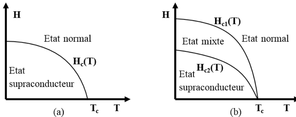
Figure I.11 Différents états en fonction de l'intensité du champ magnétique appliqué et de la température du supraconducteur, (a) type I (b) type II.
