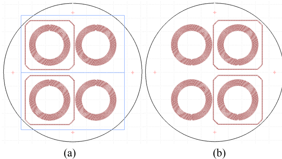
Figure III.46 Masques utilisés pour la fabrication du réseau SHTc. Ces masques comportent les motifs pour la fabrication de deux réseaux identiques. Les lignes bleues représentent les lignes de coupe. (a) face devant (b) face arrière.
