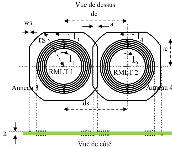
Figure III.43 Géométrie du réseau de deux RMLTs supraconducteurs. Les paramètres des RMLTs sont : rayon externe r_c , nombre de tours N , largeur de piste w_r , espacement entre pistes e , épaisseur du substrat h , distance entre RMLTs d_c . Les paramètres des anneaux sont: rayon externe r_s , largeur de piste w_s , distance entre anneaux d_s = d_c . Le niveau de chevauchement est représenté par la distance a .
