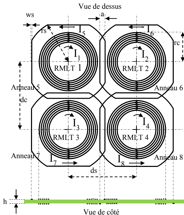
Figure III.36 Géométrie du réseau de quatre RMLTs. Les paramètres des RMLTs sont: rayon externe r_c , nombre de tours N , largeur de piste w_r , espacement entre pistes e , épaisseur du substrat h , distance entre RMLTs d_c . Les paramètres des anneaux sont: rayon externe r_s , largeur de piste w_s , distance entre anneaux d_s = d_c . Le niveau de chevauchement est représenté par la distance a .
