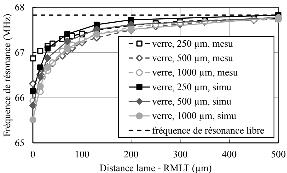
Figure II.15 Fréquences de résonance mesurée (lignes pointillés, marqueur vides) et simulée (lignes pleines, marqueurs pleins) en fonction de la distance entre le RMLT et la lame, pour des lames de verre avec une épaisseur de 250 \mu\text{m} (carré), 500 \mu\text{m} (losange) et de 1000 \mu\text{m} (cercle).
