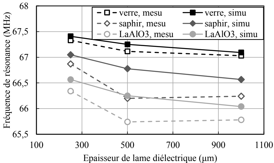
Figure II.23 Fréquence de résonance mesurée (lignes pointillées, marqueur vides) et simulée (lignes pleines, marqueurs pleins) en fonction de l'épaisseur de la lame, pour les lames de verre (carré), saphir (losange), et aluminat de lanthane (cercle), avec une distance fixée de 70 \mu\text{m} à la surface du RMLT.
