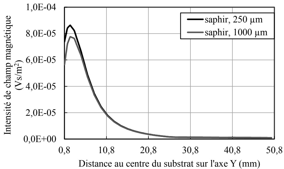
Figure II.30 Profils d'intensité du champ magnétique sur l'axe Y obtenues avec des lames de saphir de 250 \mu\text{m} et de 1000 \mu\text{m} d'épaisseurs.
