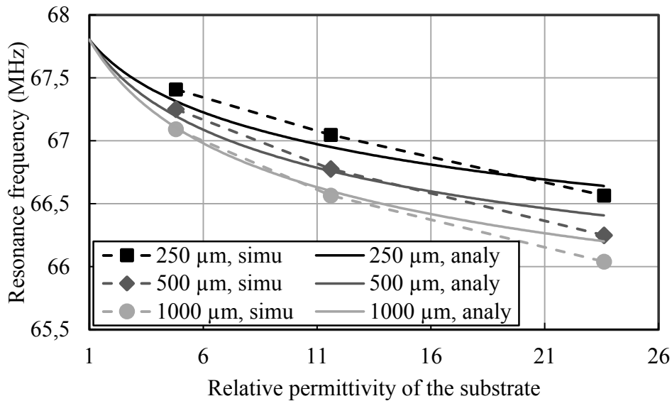
Figure II.22 Fréquence de résonance simulée (lignes pointillées, marqueurs) et calculée (lignes pleines) en fonction de la permittivité de la lame, pour les épaisseurs de lame de 250 \mu\text{m} , 500 \mu\text{m} et de 1000 \mu\text{m} , avec une distance fixée de 70 \mu\text{m} entre la lame et le RMLT.
