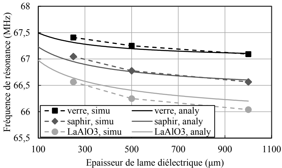
Figure II.24 Fréquence de résonance simulée (lignes pointillées, marqueurs) et calculée (lignes pleines) en fonction de l'épaisseur de la lame, pour les lames de verre (carré), saphir (losange), et aluminate de lanthane (cercle), avec une distance fixée de 70 μm à la surface du RMLT.
