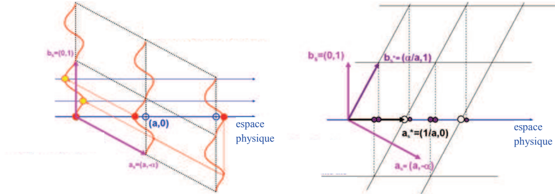
FIG. I-5: Représentation schématique d'un superspace de dimension 1+1 (a) dans l'espace réel, la courbe orange représentant la fonction atomique, la position réelle des atomes dans l'espace physique étant donnée par une coupe, (b) dans l'espace réciproque, les vecteurs de Bragg sont obtenus par projection sur l'espace réciproque physique des nœuds du superspace.
