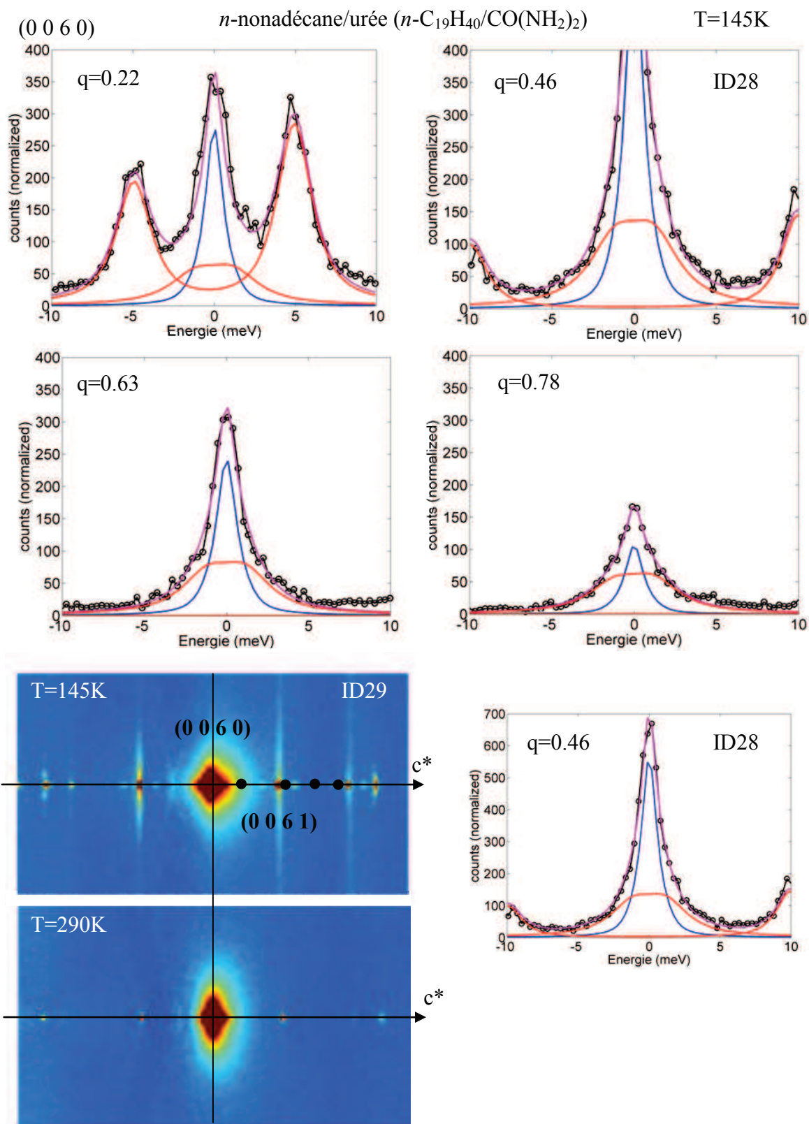
FIG V-8: Spectres en énergie du n -nonadécane/urée mesurés sur le spectromètre de ID28 à T=145K, en positions (0 0 6+ q 0), avec q =0.22, 0.46, 0.63 et 0.78 (disques noirs): pour comparaison, la même échelle en ordonnée est choisie. En bas à droite, spectre en q =0.46 à pleine échelle. En bas à gauche, images de diffraction mesurée autour de ces points à T=145K et à température ambiante sur la ligne de lumière ID29.
