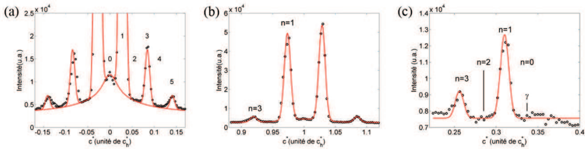
FIG III-4: Ligne de surstructure ( h=2 , k=3 ) mesurée dans la phase II du n -tétracosane/urée sur la ligne de lumière 11-3 (SSRL) (a) Autour du plan (\mathbf{a}^*, \mathbf{b}^*) en l=0 et m=0 (figure III-4a), (b) Autour d'une position du sous-réseau hôte en l=1 et m=0 (c) Autour d'une position du sous-réseau invité en l=0 et m=1 soit en position \gamma (figure III-4b). Les positions multiples du paramètre \delta ( n=0, 1, 2, \dots ) sont indiquées par des chiffres sur les figures.
