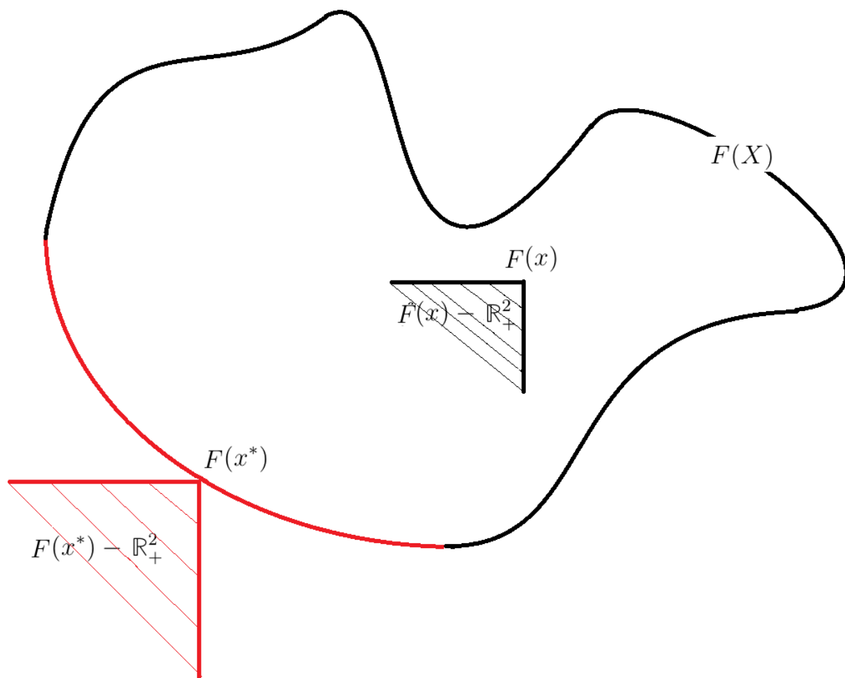
FIGURE 1.2 – En rouge, le front de Pareto \text{MIN}_{\mathbb{R}_+^2}(F(X)) de l'ensemble F(X) \subset \mathbb{R}^2
