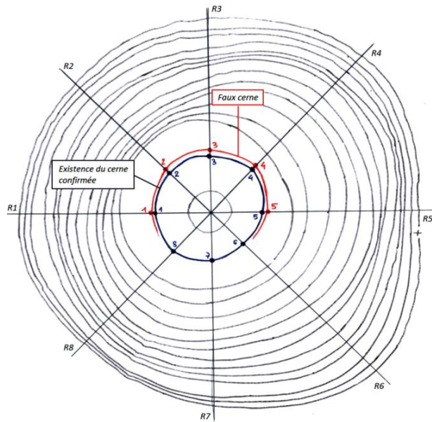
Figure 26 : Identification des cernes de croissance chez C. alliodora . Le cerne en noir est observé sur chacun des huit rayons. Son existence est donc confirmée. A l'inverse, le cerne en rouge n'est observé que sur cinq rayons. Ce dernier est considéré comme faux cerne, et ne sera pas mesuré.
