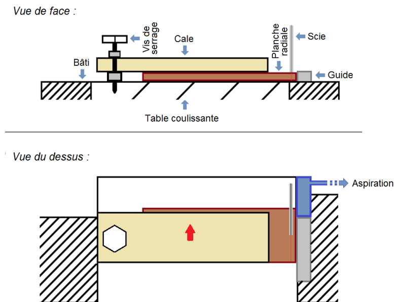
Figure 147 : Schéma du dispositif mis en place pour la découpe précise des échantillons de module. De haut en bas : vue de face et vue du dessus de la planche radiale à débiter. La planche est positionnée en butée sur le guide puis serrée sous la cale à l'aide d'une vis de serrage solidaire de la table coulissante de la scie à format. L'avancée de la table coulissante de la scie à format (dans le sens de la flèche rouge) permet la découpe de l'échantillon, aspiré en fin de processus par le système d'aspiration positionné près de la scie, en bleu sur le schéma.
