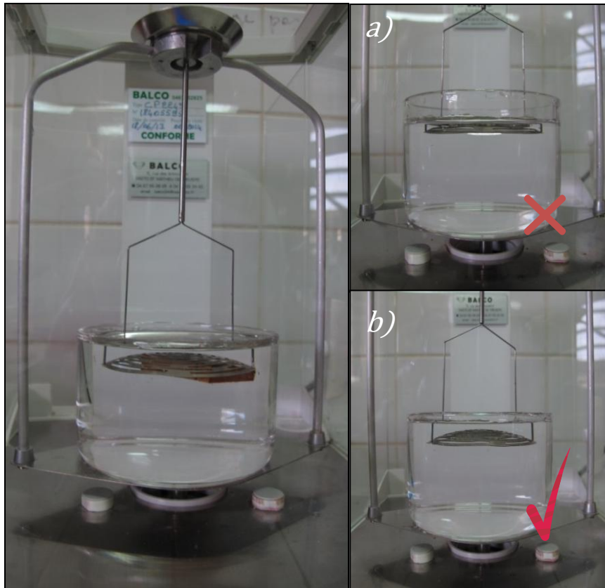
Figure 87 : Détail de la mesure du volume saturé dans le cas d'une éprouvette flottante lors de la mesure d'infradensité. L'échantillon après avoir été pesé vert est immédiatement plongé dans le béccher et positionné sous le panier de la tige reliée à la balance. Il faut veiller à ce qu'aucune bulle ne se forme entre l'échantillon et le panier, erreur qui surestime le volume saturé. a) : mauvaise utilisation du dispositif ; b) : mesure correctement effectuée
