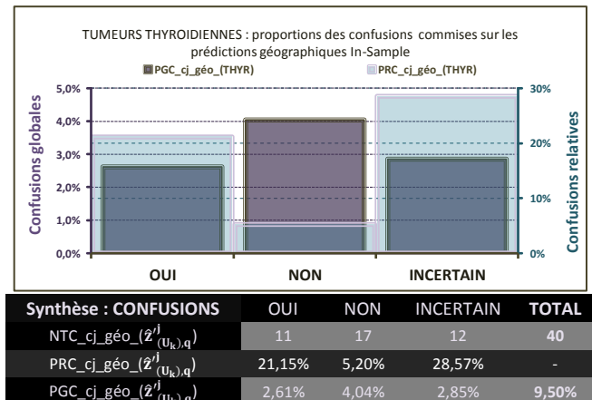
Figure 242 : Synthèse et représentation graphique des \zeta_{(U_k)}^{THYR}
