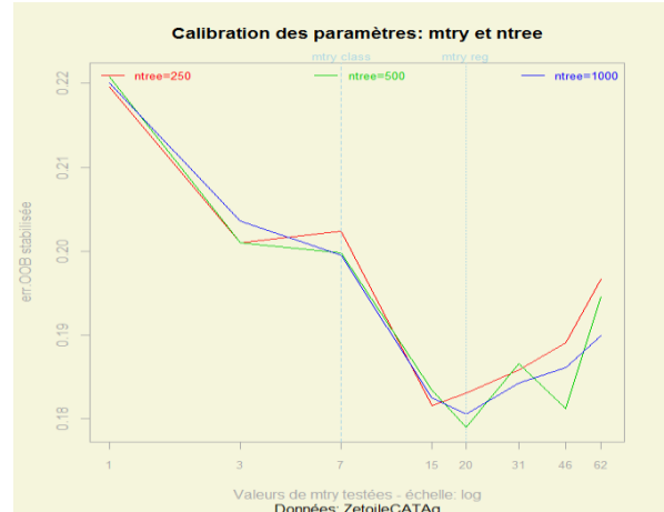
Figure 205 : \bar{R}^{OOB}(\cdot) en fonction de ntree et mtry
