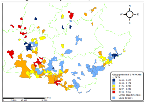
Variabilité spatiotemporelle des émissions radioactives globales des particules \beta dans l'eau
