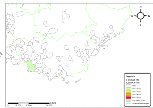
Figure 141 : Superposition des \mathfrak{Z}_{(U_k)}^{(r_j=0m)} et des x_{(U_k)}^{EGRA} (r_j=0m)
