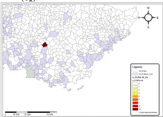
Figure 140 : superposition des x_{(U_u)}^{EGRA.R_0} des U_k et des \mathfrak{Z}_{(U_k)}^{(r_j=0m)}
