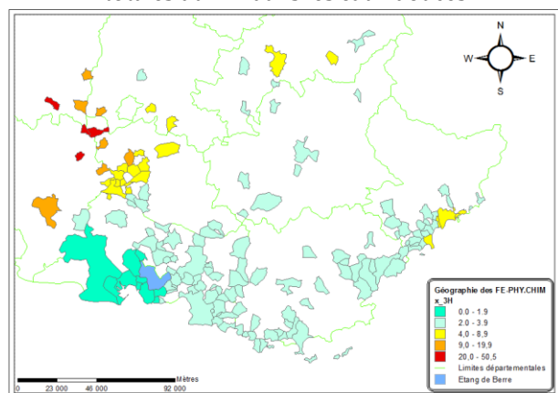
Variabilité spatiotemporelle des émissions radioactives totales du ^3H dans les eaux douces
