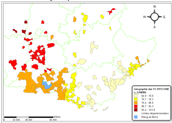
Variabilité spatiotemporelle des émissions globales des rayons \gamma dans l'air ambiant
