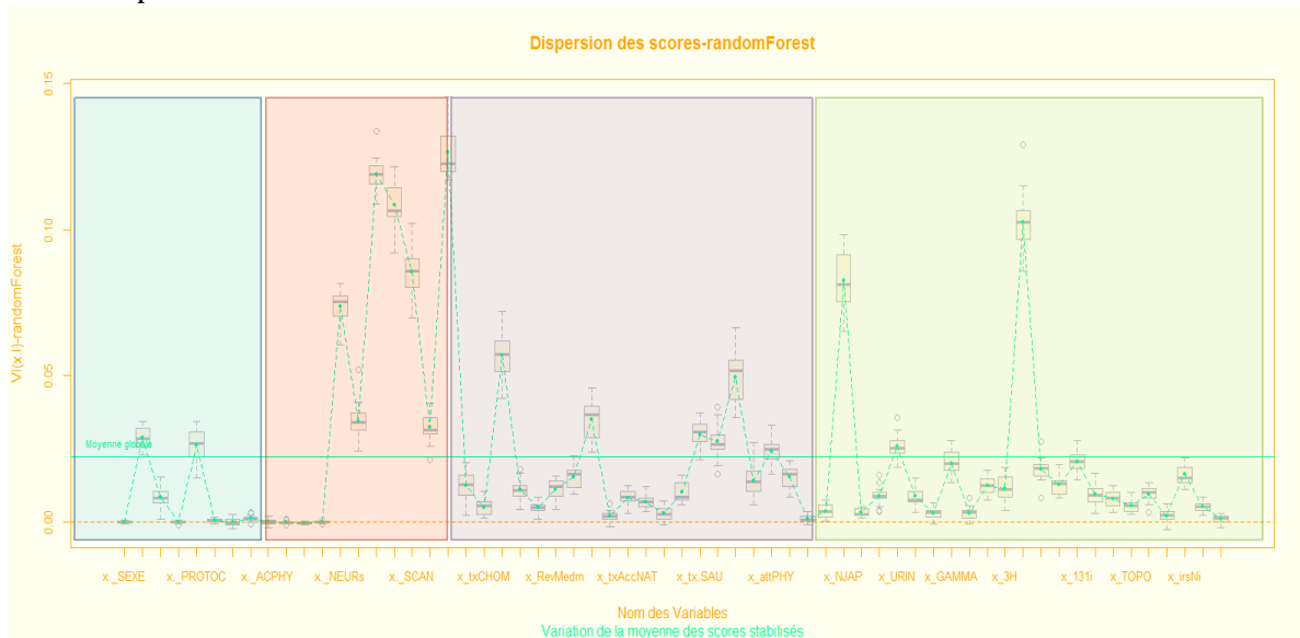
Figure 258 : Diagramme de Tukey des V_{j,r}(z^j_{(.)}) , \bar{V}_j(z^j_{(.)}) et \bar{V}_j(z^j_{(.)}) - estimation stabilisée sur 50 forêts.
