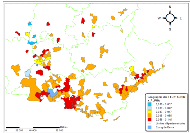
Variabilité spatiotemporelle des émissions radioactives globales des particules \alpha dans l'eau
