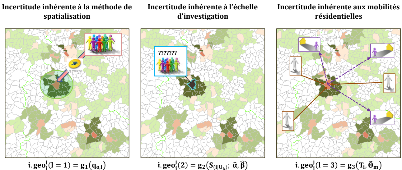
Figure 25 : Synoptique d'estimation du facteur d'incertitude spatiotemporelle à connotation géographique
