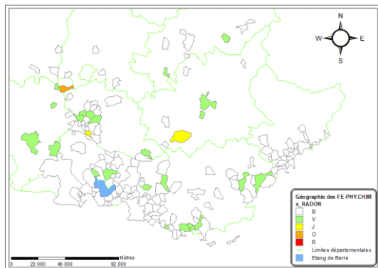
Variabilité de l'Activité Volumique du Radon dans les habitations
