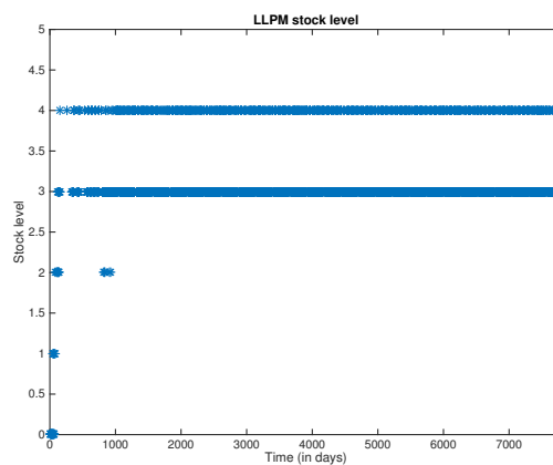
FIGURE 6.2 – Évolution du stock de SRM dans le temps pour la vitesse maximale de production
