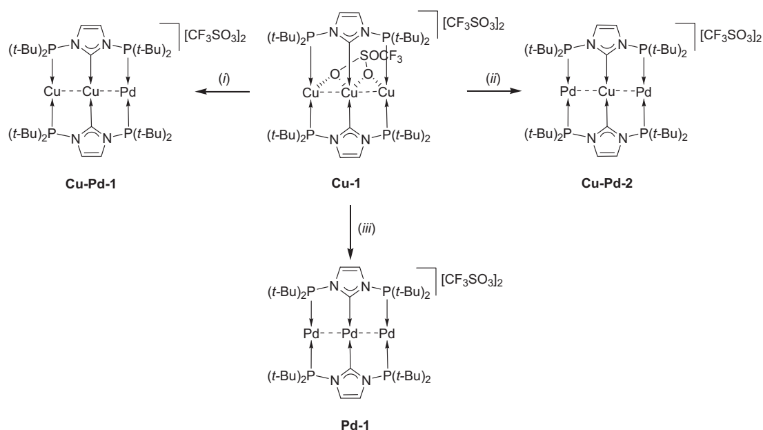
Schéma 1. Réactions de transmétallation du complexe trinucléaire Cu-1 . Réactifs et conditions: (i) 1.2 equiv [Pd(PPh 3 ) 4 ], CH 2 Cl 2 , 12 h, temp. amb.; (ii) 3 equiv [Pd(PPh 3 ) 4 ], CH 2 Cl 2 , 12 h, temp. amb.
