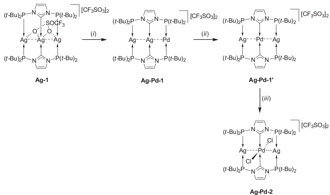
Schéma 2. Réactions de transmétallation du complexe trinuécléaire Ag-1 . Réactifs et conditions: (i) 1 equiv [Pd(PPh_3)_4] , CH_2Cl_2 , 1 h, temp. amb.; (ii) évaporation lente et complète à l'air; (iii) solide laissé dans MeCN/CH_2Cl_2 (10:1) pendant deux semaines à temp. amb.
