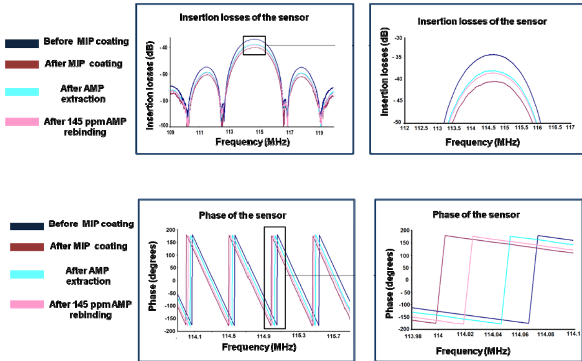
Figure V. 1 Pertes d'insertion et réponse en phase du capteur pour une concentration de 145 ppm d'AMP.
