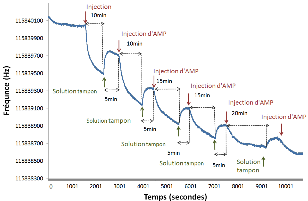
Figure V. 16 Recaptures successives d'une solution d'AMP à une concentration de 300 ppm jusqu'à saturation.
