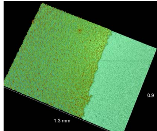
Figure IV. 18 Caractérisation par profilométrie optique a) profil 2 D du bord de la couche mince de MIP/AMP sur le capteur (230, vitesse 2200 rpm), b) image 3 D de surface.
