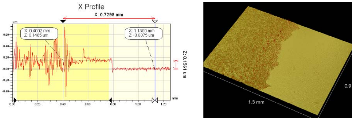
Figure IV. 16 Caractérisation par profilométrie optique a) profil 2 D du bord de la couche mince de MIP/AMP sur le capteur (34 nm, vitesse 2500 rpm), b) image 3 D de surface.
