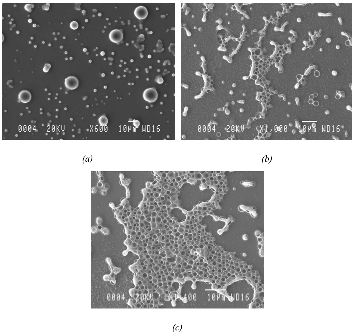
Figure IV. 24 Clichés MEB de couches MIP-DMSO déposées sur des capteurs avant extraction de la molécule empreinte en fonction du temps de mélange de la solution MIP: a) 1h, b) 3h et c) 6h.
