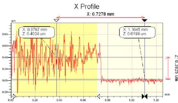
Figure IV. 18 Caractérisation par profilométrie optique a) profil 2 D du bord de la couche mince de MIP/AMP sur le capteur (230, vitesse 2200 rpm), b) image 3 D de surface.
