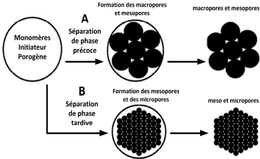
Figure IV. 23 Représentation schématique de la structure macroporeuse d'un MIP selon la nature du porogène, A) porogène à faible pouvoir solvatant, B) porogène à fort pouvoir solvatant (N. Omar-Aouled, 2013) adaptée de (M. H. Mohamed et al., 2012).
