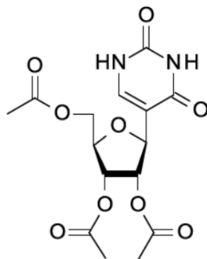
Figure IV. 29 Structure chimique de 2',3',5'-O-triacetyl-uridines, molécule analogue du nucléoside pseudouridine
