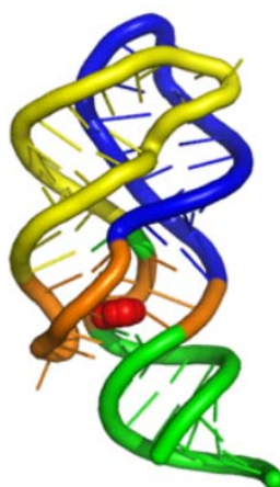
Figure I. 8 Structure d'un aptamère
