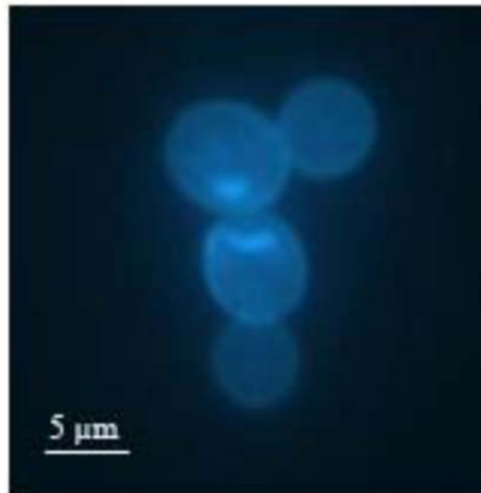
Figure II. 5 Image obtenue par microscopie fluorescente d'une cellule de levure ( S. cerevisiae ) en phase S marquée par du fluorochrome bisbenzimidazole (Seidler et al., 2009).
