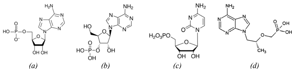
Figure V. 18 Nucléotides utilisées pour les tests de recapture en temps réel: (a) adénosine-5'-monophosphate, (b) adénosine-3'-monophosphate (c) cytidine-5'-monophosphate, (d) 2-phosphonométhoxypropyladénine.
