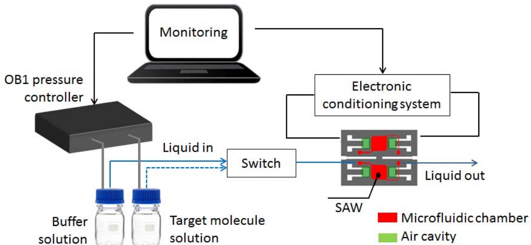
Figure III. 17 Description du banc de mesure pour la détection d'AMP en temps réel
