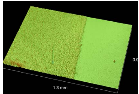
Figure IV. 19 Caractérisation par profilométrie optique a) profil 2 D du bord de la couche mince de MIP/AMP sur le capteur (380 nm, vitesse 2100 rpm), b) image 3 D de surface.
