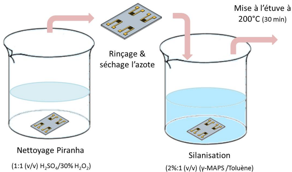
Figure IV. 4 Représentation des étapes de traitement de surface des substrats avant le dépôt des couches de MIP
