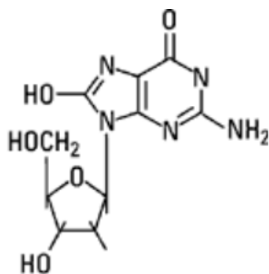
Figure IV. 34 Structure chimique du biomarqueur 8-hydroxy-2'deoxyguanosine (8-OHdG) www.sigmaaldrich.com .
