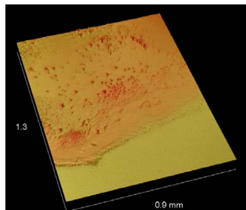
Figure IV. 20 Caractérisation par profilométrie optique a) profil 2 D du bord de la couche mince de MIP/AMP sur le capteur (500 nm, vitesse 2000 rpm), b) image 3 D de surface.
