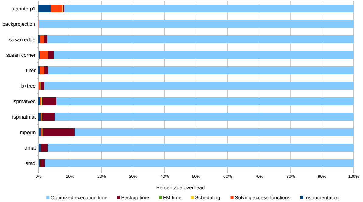
Figure 9: Classification des surcoûts temporels en pourcentages
