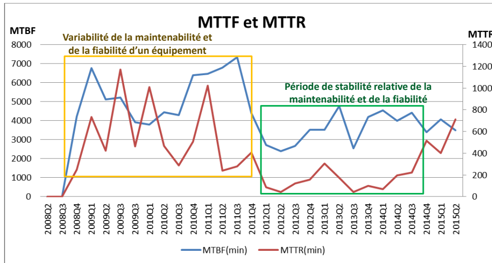
Figure I 12 Variabilité de la maintenabilité et de la fiabilité
