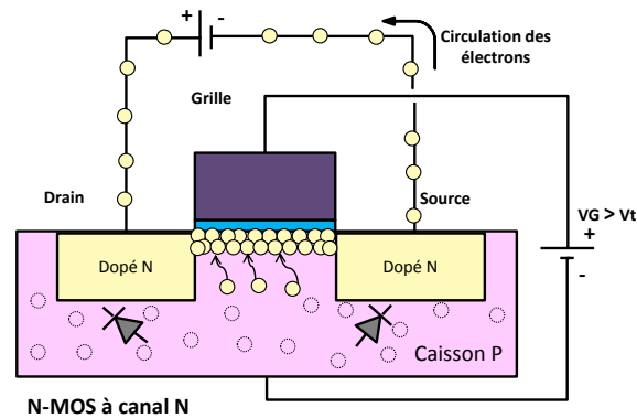
Figure I 2 Principe de fonctionnement du transistor MOS à canal N (NMOS) (Micolet, 1987)
