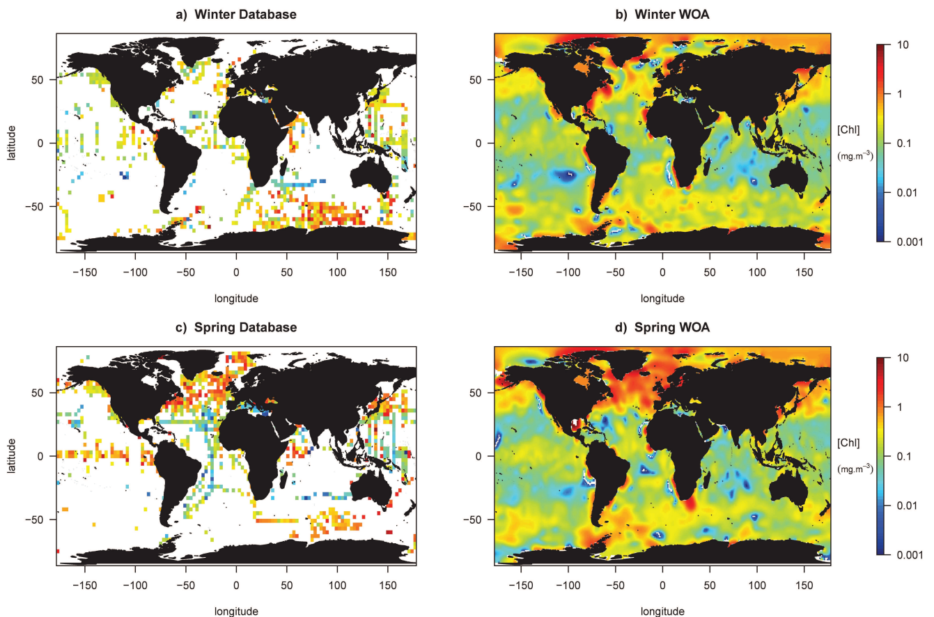
FIGURE 2.2 – Comparaison des données climatologiques saisonnières de surface provenant de BD-FLAVOR (i.e. base de données calibrée) moyennées dans des mailles de 3^{\circ} \times 3^{\circ} avec les climatologies saisonnières provenant du WOA pour : a) et b) l'hiver (mois de janvier, février et mars) et c) et d) le printemps (mois d'avril, mai et juin).
