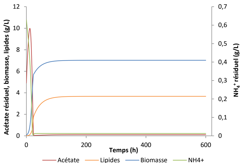
Figure V- 9. Simulation d'une culture continue de C. curvatus .
