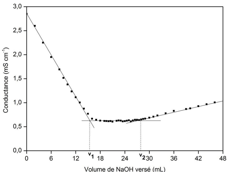
Figure 94 : Courbe de titration par conductimétrie de l'écorce Ebrute.
