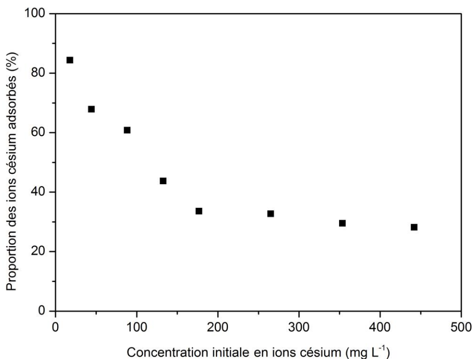
Figure 30 : Proportion des ions césium adsorbés sur l'écorce Ecburte en fonction de la concentration initiale. Conditions opératoires : T = 25 °C ; 100 mg d'écorce ; V = 50 mL ; temps de contact = 2 h ; pH = 5,6.
