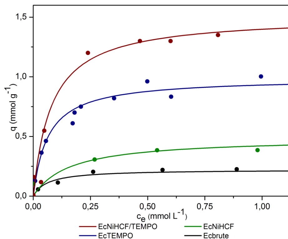
Figure 45 : Isothermes d'adsorption des ions césium par les écorces Ecbrute, EcNiHCF, EcTEMPO et EcNiHCF/TEMPO. Conditions opératoires : T = 25 °C ; 100 mg d'écorce ; V = 50 mL ; [Cs^+]_0 = 0 - 700 mg L -1 ; pH = 5,6 ; temps de contact = 2 h.
