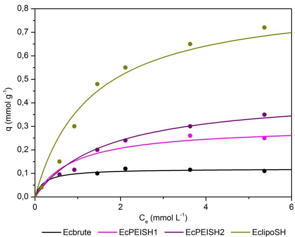
Figure 93 : Isothermes d'adsorption de l'As(III) par les écorces Ecrute, EcPEISH1, EcPEISH2 et EclipoSH. Conditions opératoires : T = 25\text{ }^\circ\text{C} ; 100 mg d'écorce ; V = 50\text{ mL} ; \text{pH} = 5 ; temps de contact = 2 h ; [\text{As(III)}] = 0\text{-}700\text{ mg L}^{-1} .
