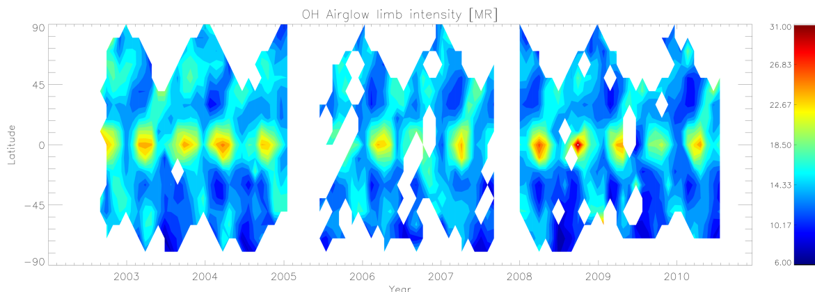
FIGURE 3.15 – De manière similaire à la figure 3.11, l'évolution de l'émission OH entre 2002 et 2010. Très nettement apparaissent les pics d'émission au niveau de l'équateur d'une périodicité semi-annuelle. Aux latitudes moyennes, l'émission tend progressivement vers une variation annuelle avec le maximum aux solstices.
