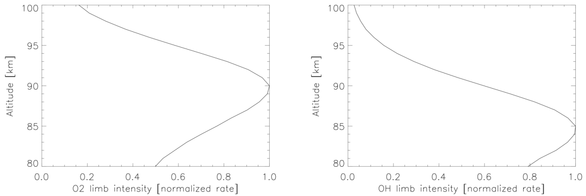
FIGURE 3.13 – Profils verticaux moyennés des émissions O_2 (à gauche) et OH (à droite). L'altitude du maximum varie selon l'espèce : elle est de 90 km pour O_2 et 85 pour OH . Elle varie également selon les latitudes considérées (voir figure 3.14).
