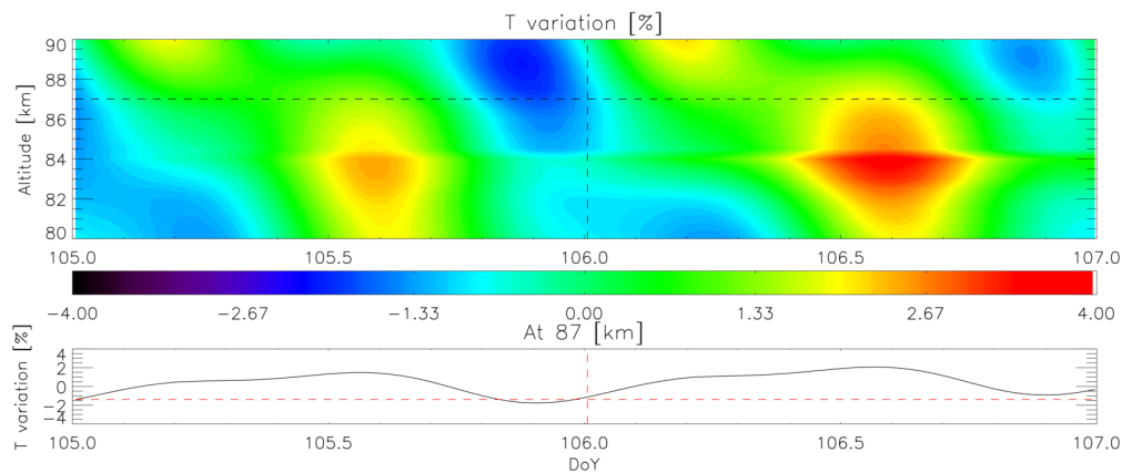
FIGURE 7.24 – Variation relative de température entre le cas de l’itération normale et le cas de l’itération sans dynamique, selon (T_{\text{normal}} - T_{\text{cas}})/T_{\text{normal}} . La variation diurne induite par les marées apparaît également, en opposition de phase par rapport à la densité, représentée dans la figure 7.23.
