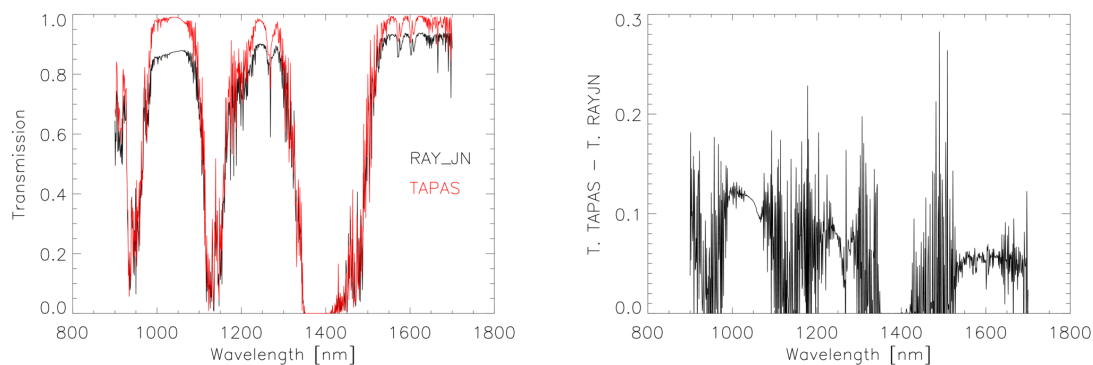
FIGURE 5.14 – À gauche, zoom sur la bande spectrale comprise entre 900 et 1700 nm. L’absorption autour de 1.4\ \mu\text{m} provient de la vapeur d’eau. La différence entre les transmissions TAPAS et RAYJN s’observe nettement entre 1. et 1.1\ \mu\text{m} , mais s’estompe dès 1.3\ \mu\text{m} , ce qui s’explique par l’absence des aérosols dans TAPAS. À droite est représentée la différence entre RAYJN et TAPAS.
