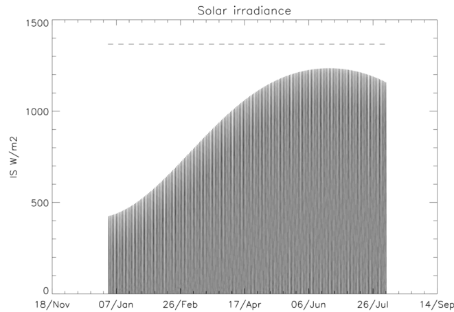
FIGURE 5.3 – Évolution de l'irradiance solaire au cours du temps, pour une latitude de 45^\circ\text{N} sur 7 mois. En traits pointillés est représentée l'irradiance solaire maximale à 1367 \text{ W/m}^2 .
