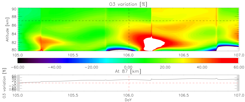
FIGURE 7.22 – Variation relative de \text{O}_3 entre le cas de l’itération normale et le cas de l’itération sans chauffage, selon ([\text{O}_3]_{\text{normal}} - [\text{O}_3]_{\text{cas}}) / [\text{O}_3]_{\text{normal}} . On observe ici une correspondance forte entre l’évolution de la concentration de l’ozone et l’évolution du VER (figure 7.21).
