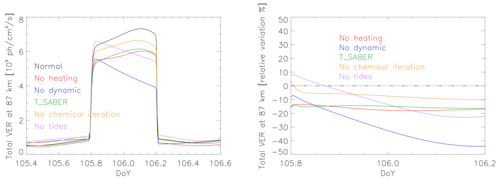
FIGURE 7.16 – Comparaisons de l'évolution du VER total à 87 km d'altitude. En noir correspond l'itération normale, en rouge, en l'absence de chauffage, en bleu, en l'absence de dynamique, en vert, avec la température issue des données SABER et en orange, sans l'itération chimique. La comparaison à gauche est en valeur absolue, et à droite en variation relative par rapport à l'itération normale.
