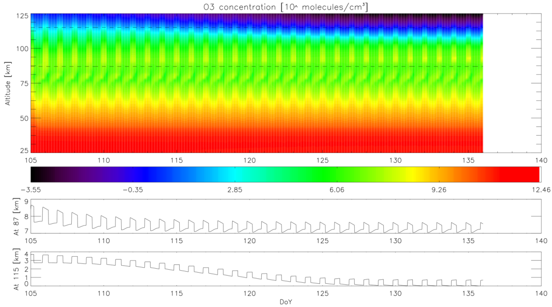
FIGURE 5.18 – Évolutions de la concentration en ozone sur 30 jours en \text{molécules/cm}^3 (échelle logarithmique) pour le modèle photochimique 0D réparti sur une grille d'altitude 1D. L'abscisse correspond au jour de l'année ( DoY pour Day of Year ). Si l'ensemble est assez stable, on observe une augmentation du gradient de concentration au dessus de 115 km qui peut conduire à une divergence sur des durées plus longues.
