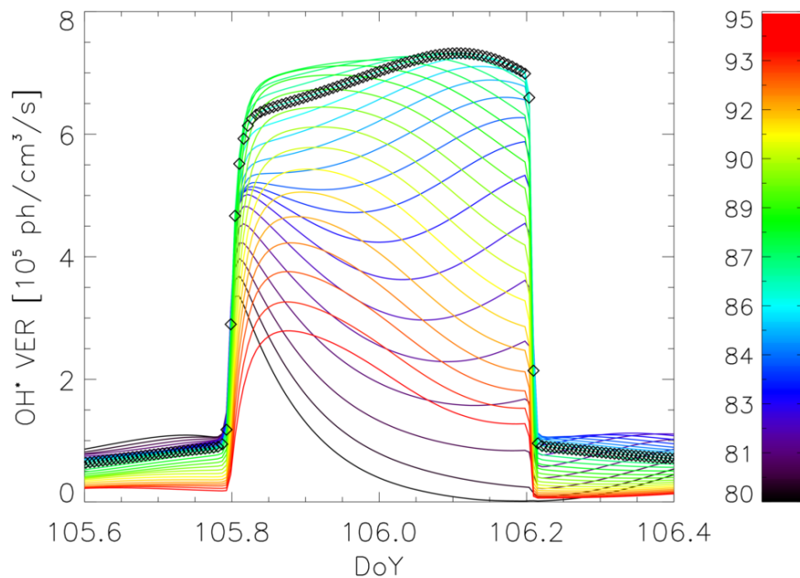
FIGURE 7.12 – Évolution du VER total sur une nuit, selon les altitudes, représentées par la barre de couleur. En losange, l'altitude de 87 km est superposée. On constate que l'évolution du rayonnement est différente selon l'altitude que l'on considère.
