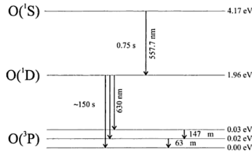
FIG. 3.3 – Niveaux d'énergie de l'atome d'oxygène.
