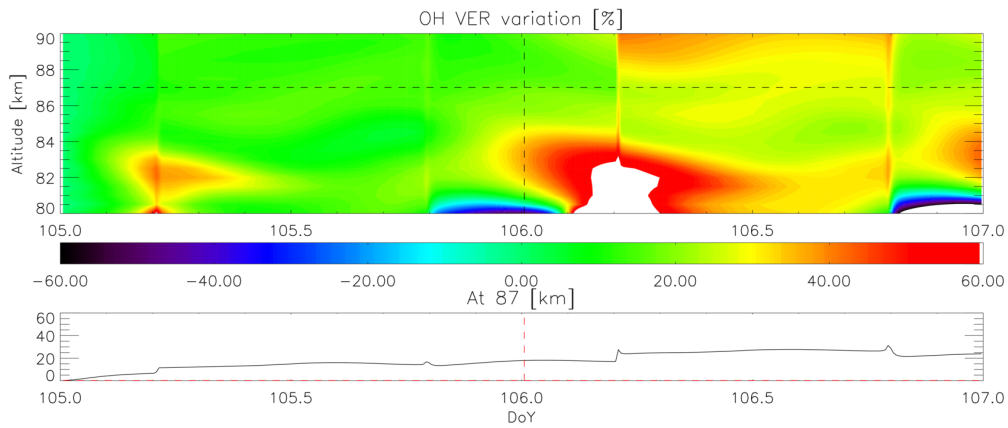
FIGURE 7.21 – Variation relative de l’émission totale de \text{OH}^* entre le cas de l’itération normale et le cas de l’itération sans chauffage, selon (\text{VER}_{\text{normal}} - \text{VER}_{\text{cas}}) / \text{VER}_{\text{normal}} . L’évolution du VER ne suit pas celle de la température observée dans la figure 7.20.
