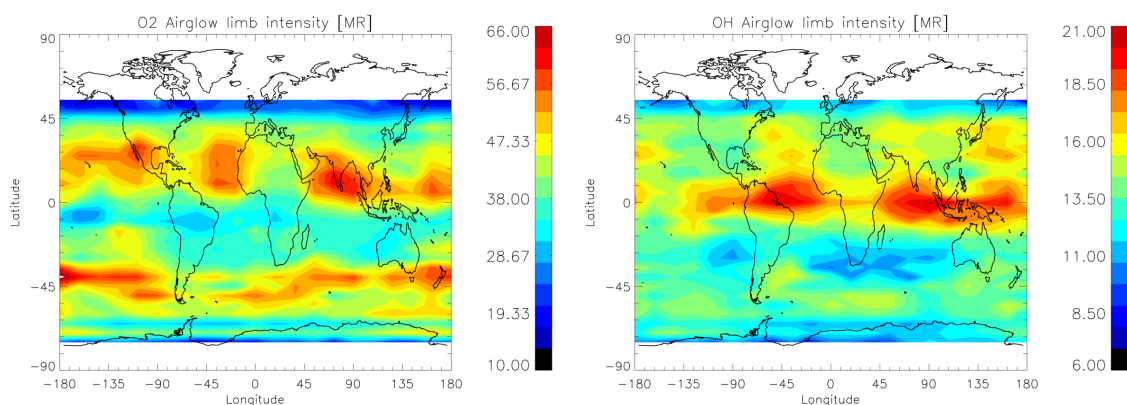
FIGURE 3.16 – Émission du rayonnement O_2 (à gauche) et OH (à droite). Les valeurs correspondent à une moyenne des mois d'avril, mai et juin. Des maxima d'émission sont présents à des longitudes similaires, pour O_2 entre 0^\circ et 45^\circ , pour OH autour de l'équateur.
