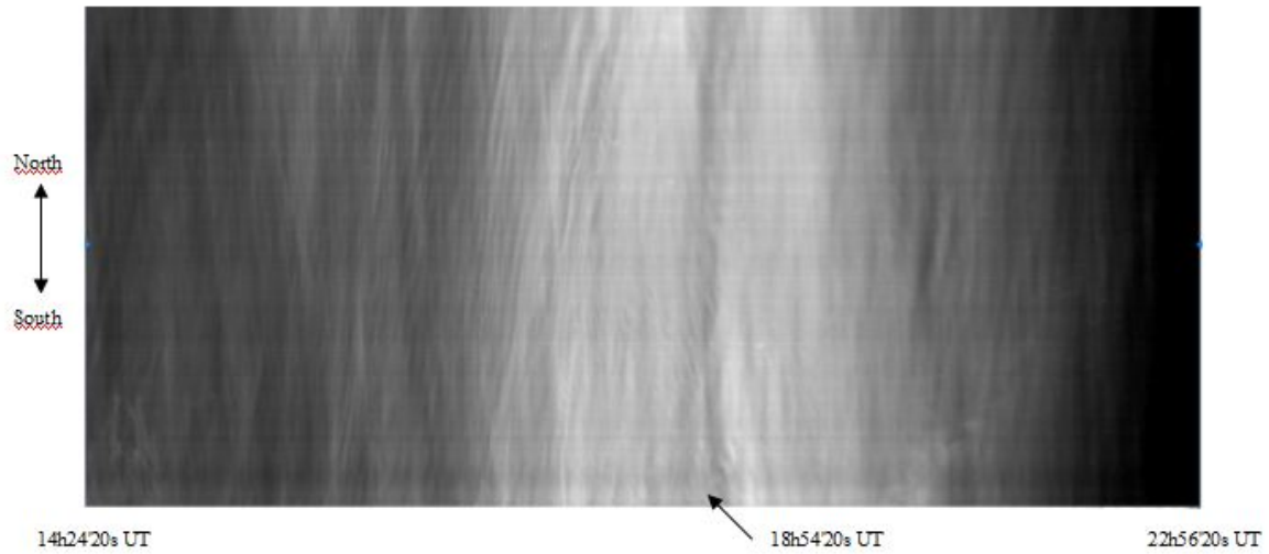
FIGURE 4.20 – Kéogramme obtenu à partir de chaque image de la vidéo, bande mesurant 150 \times 0.2 km. Au milieu apparaît la chute d'intensité observée sur les figures 4.19.
