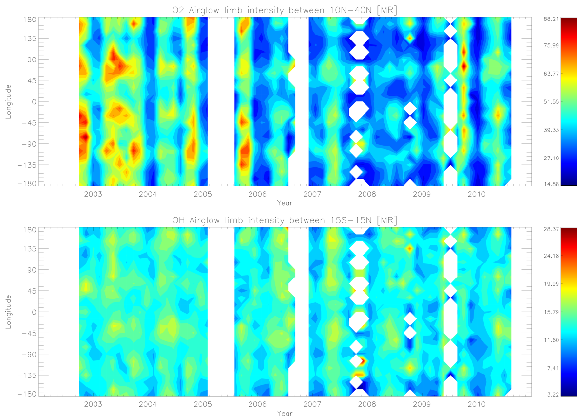
FIGURE 3.17 – Évolution du rayonnement O_2 (haut) et OH (bas) selon les longitudes entre 2002 et 2010. Les latitudes considérées ici sont comprises entre -15^\circ et 15^\circ pour OH, 10^\circ et 40^\circ pour O_2 . On remarque une chute de l'intensité globale de O_2 mesurée au cours du temps avec un minimum entre 2008 et 2009.
