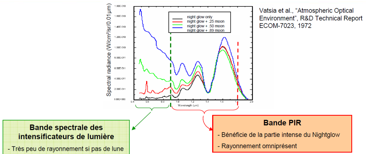
FIGURE 1.6 – Éclairement spectral pour différents types de nuit adaptée de Vatsia [1972] selon la fraction de Lune visible. Deux bandes spectrales sont observées : l'une dans le visible utile aux intensificateurs de lumière, et l'autre dans la bande Proche InfraRouge (PIR). On observe la continuité de la disponibilité dans la bande PIR correspondant à l'émission du nightglow.
