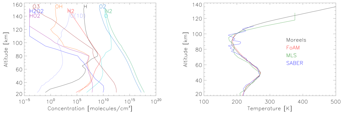
FIGURE 5.1 – Exemple de données initiales utilisées, tirées moyennes journalières de Moreels et al. [1977]. On remarque la prédominance de \text{N}_2 et \text{O}_2 , constituant à eux deux plus de 98% de l'atmosphère. À droite, quelques profils de température, correspondant à des profils standards [Jacobson, 2005; Moreels et al., 1977], mais aussi correspondant à des données satellitaires, MLS et SABER.
